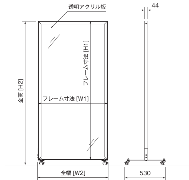
900×1800サイズ キャスター仕様 シルバー
