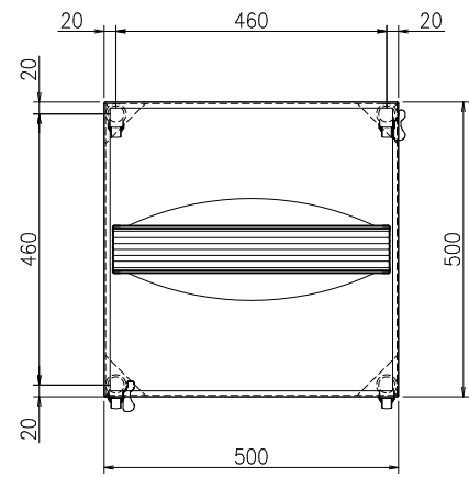
上面姿図(1:10)
