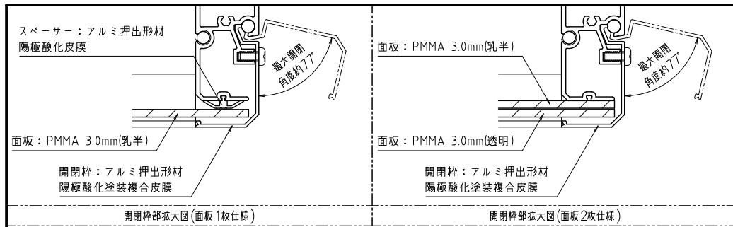
開閉枠部拡大図(面板1枚仕様)
