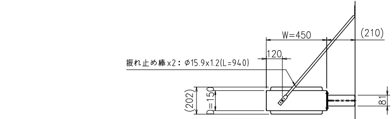
上面側姿図 1:20
