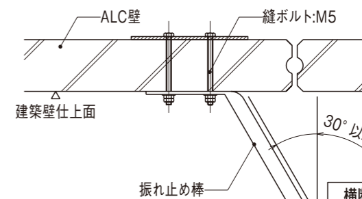
横断面詳細図
