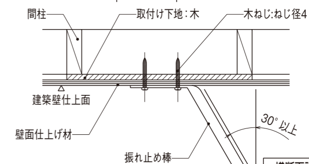
横断面詳細図
