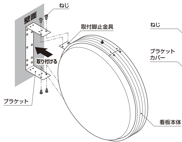
ブラケットの孔位置について
