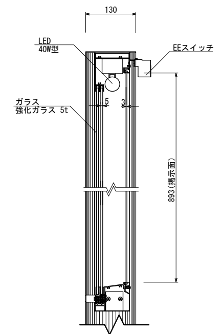
【側断面図 S=1:10】
