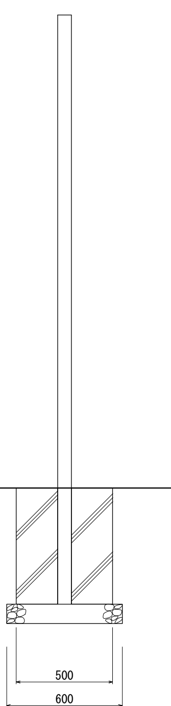
【側面図 S=1/20】
