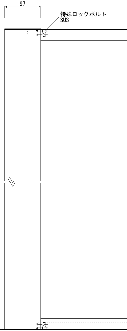
【正面図 S=1:5】
