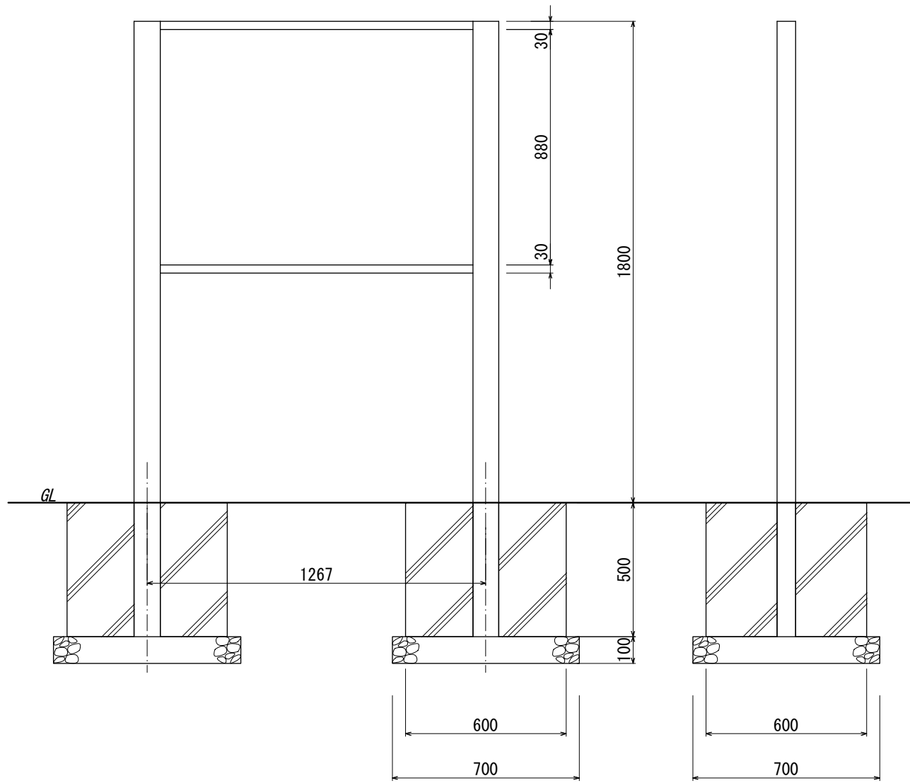
【正面図 S=1:20】
