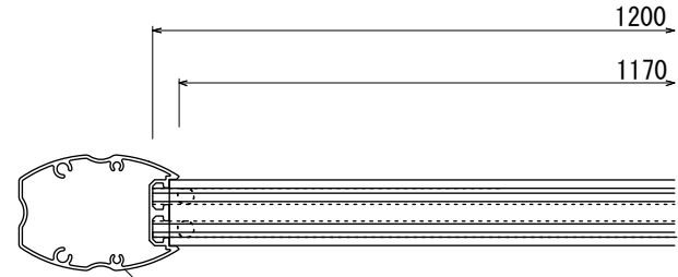
【平面図 S=1:5】
