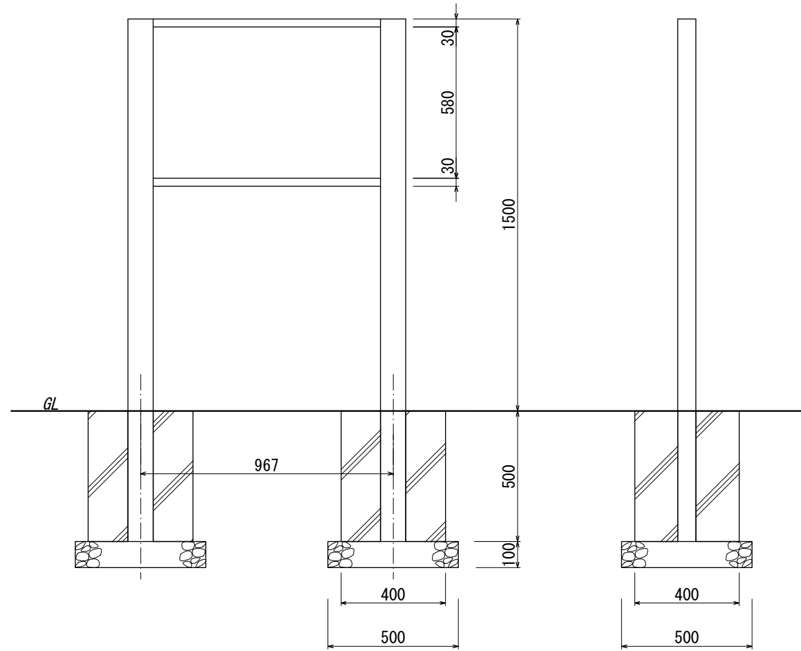
【正面図 S=1:20】
