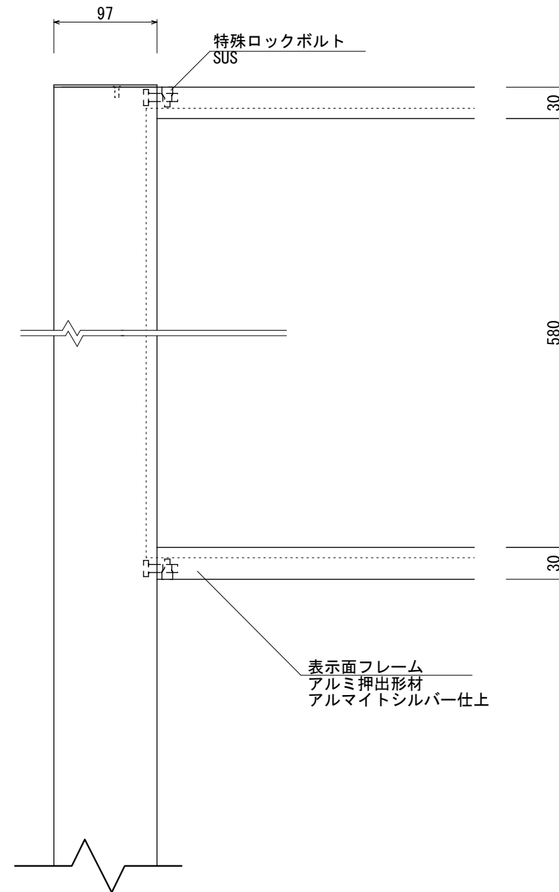
【正面図 S=1:5】
