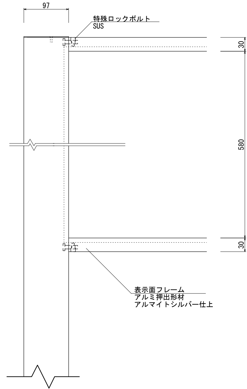
【正面図 S=1:5】
