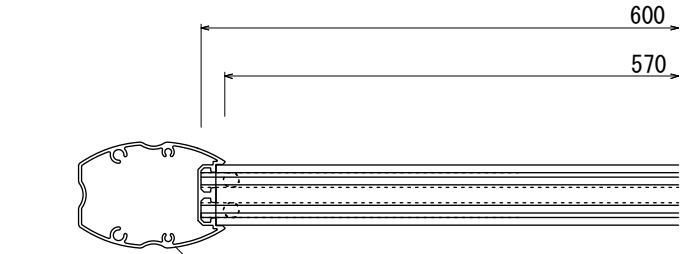
【平面図 S=1:5】
