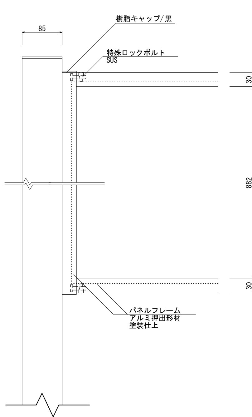
【正面図 S=1:5】
