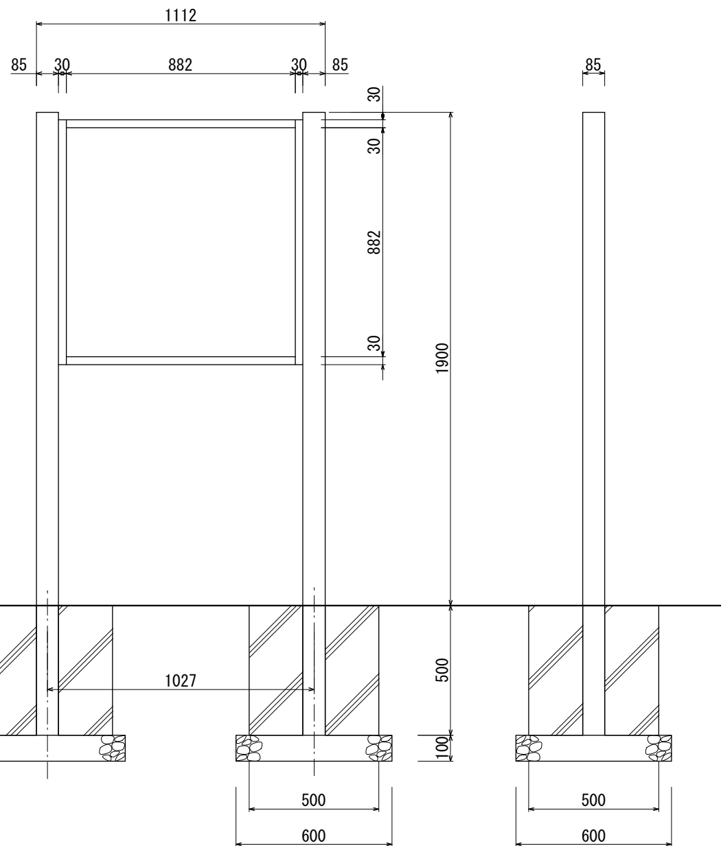
【正面図 S=1:20】
