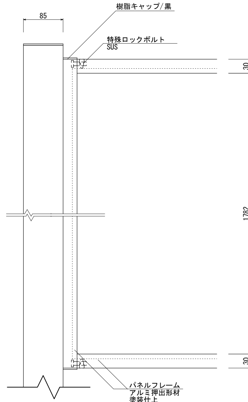
【正面図 S=1:5】
