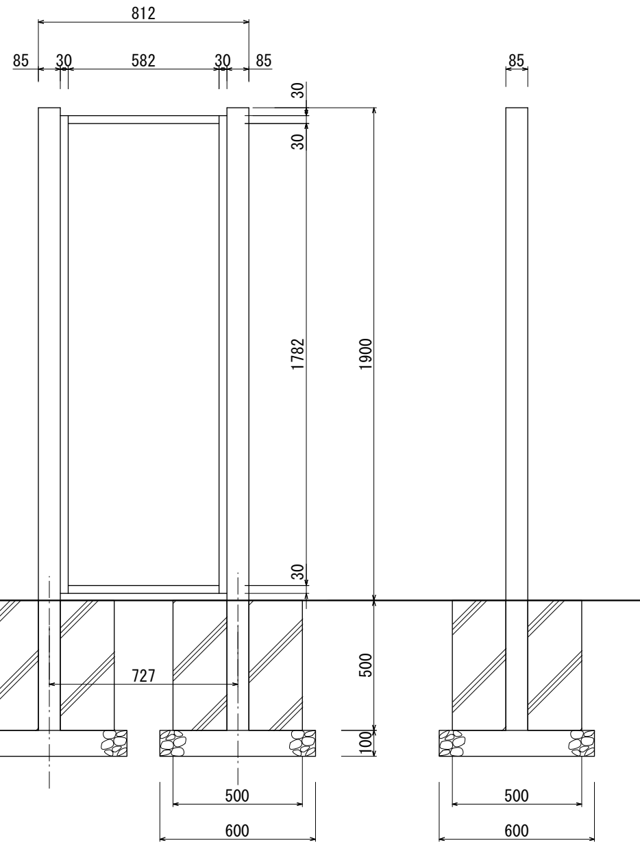
【正面図 S=1:20】
