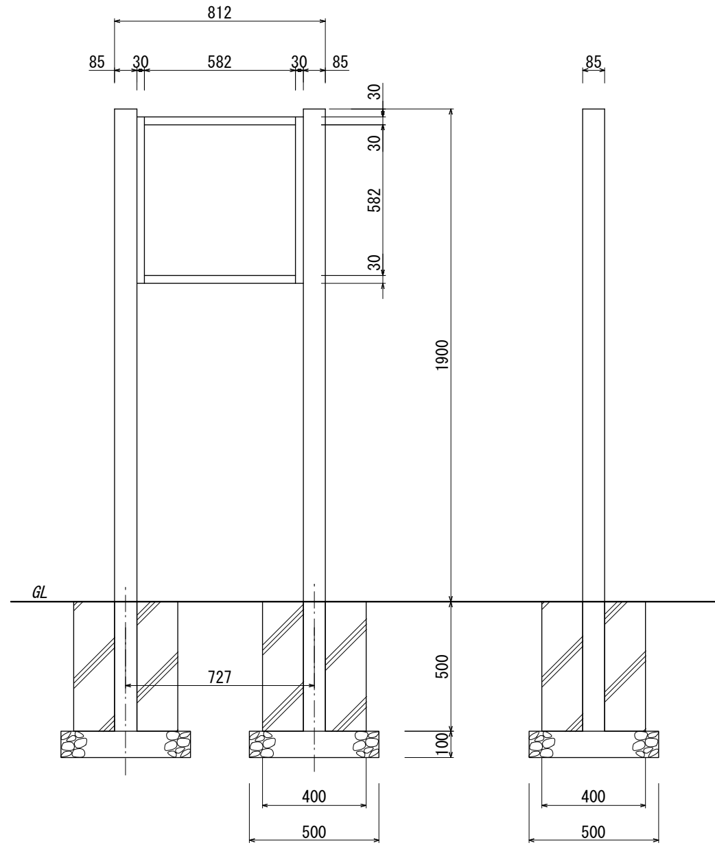
【正面図 S=1:20】
