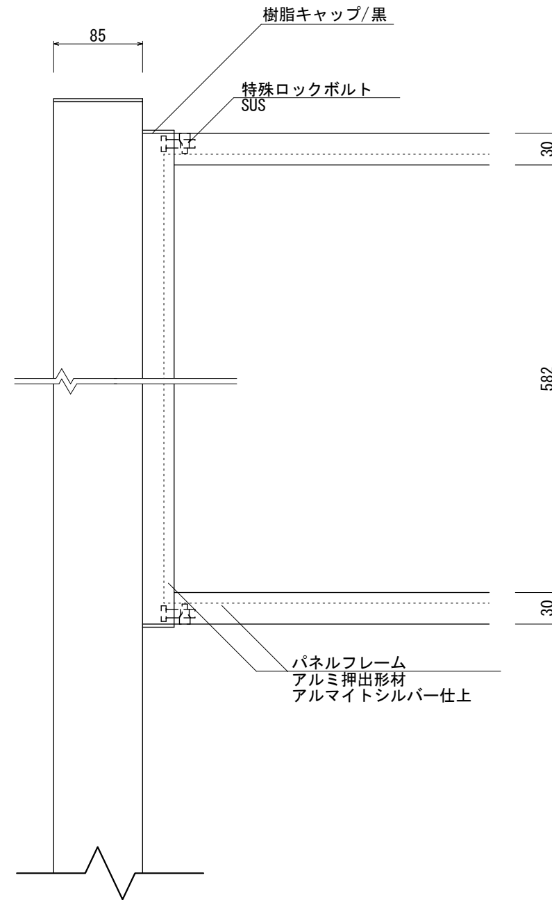
【正面図 S=1:5】
