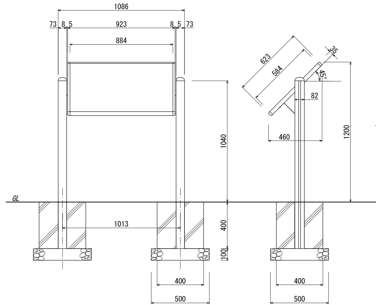
【正面図 S=1:20】
