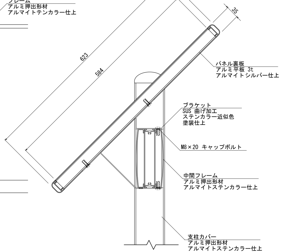
【側断面図 S=1:5】
