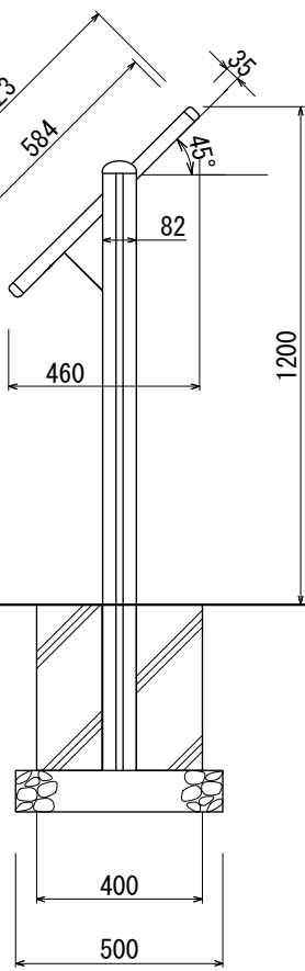
【側面図 S=1:20】
