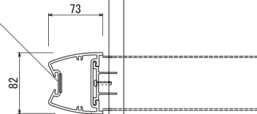
【平面図 S=1:5】
