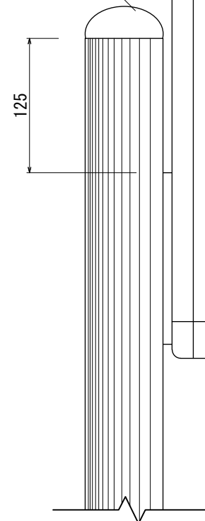
【正面図 S=1:5】
