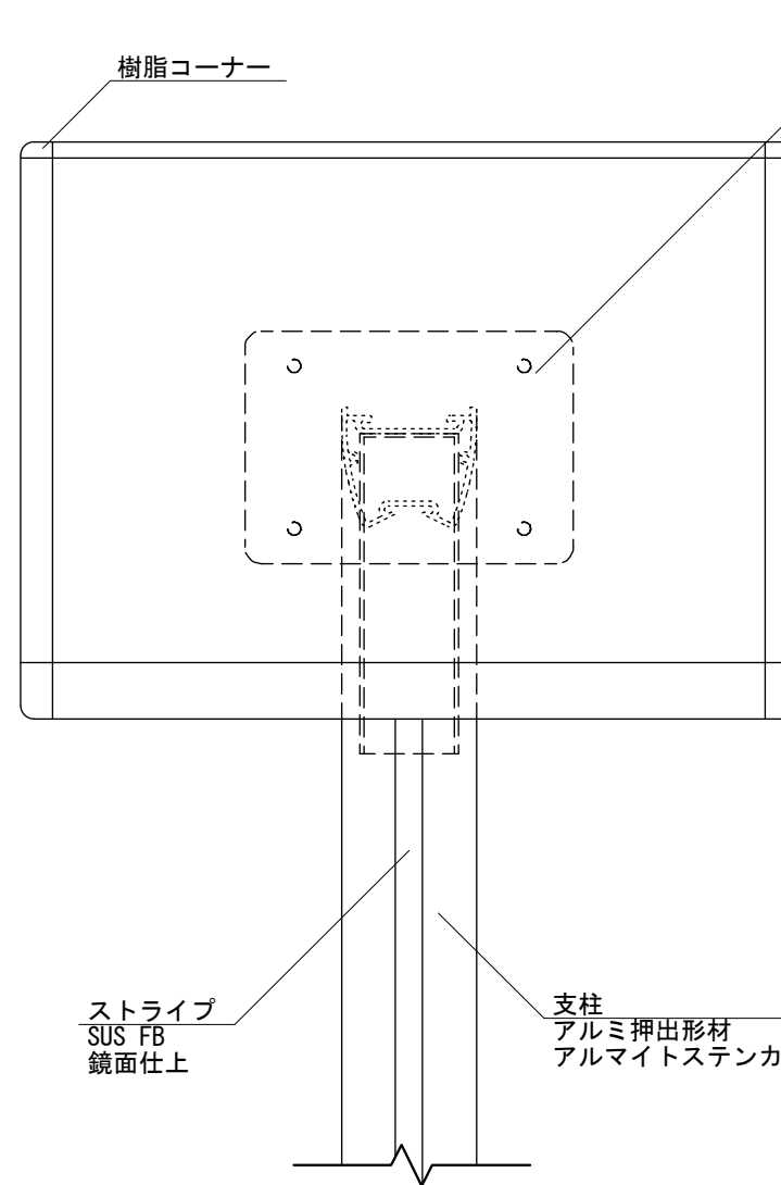
【正面図 S=1:5】
