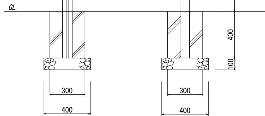
【正面図 S=1:20】
