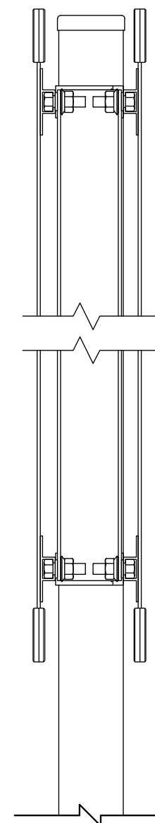
【側面図 S=1:5】
