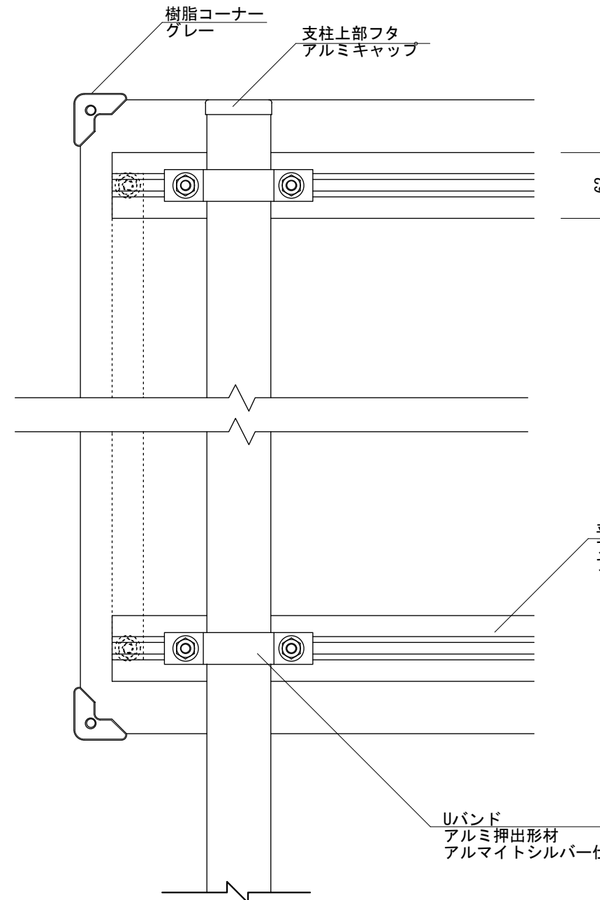
【背面図 S=1:5】
