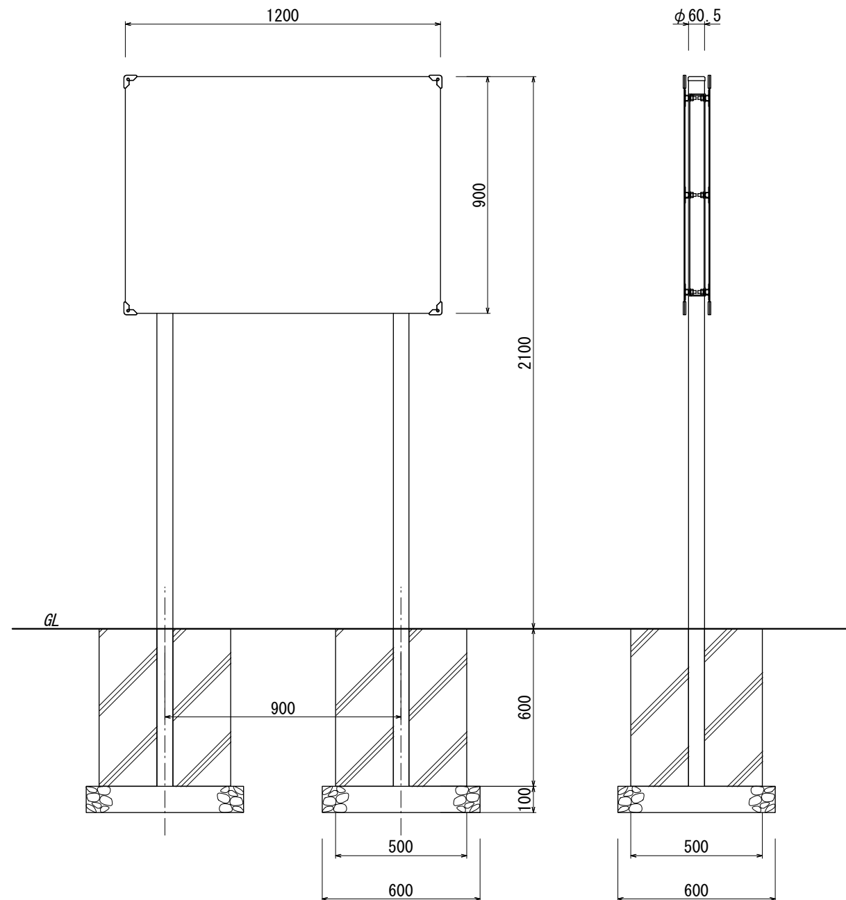
【正面図 S=1:20】
