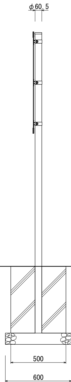
【側面図 S=1:20】
