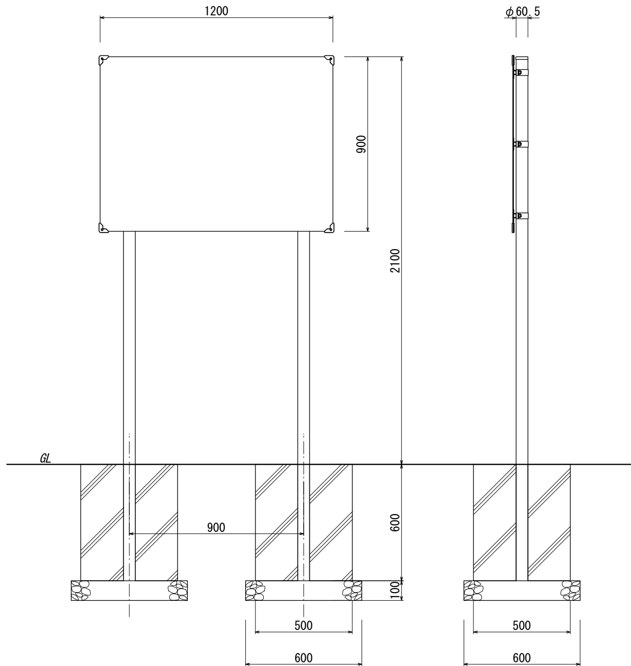
【正面図 S=1:20】
