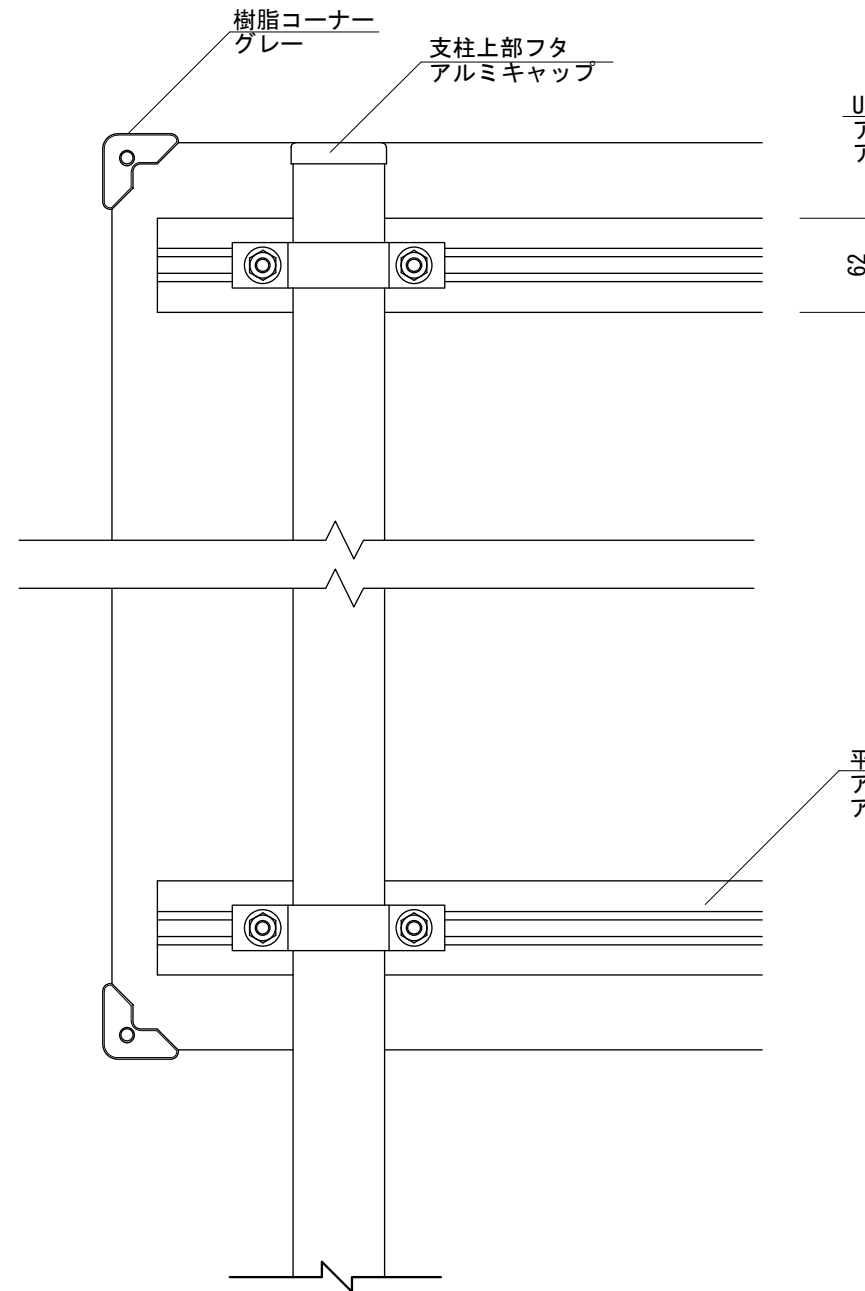
【背面図 S=1:5】
