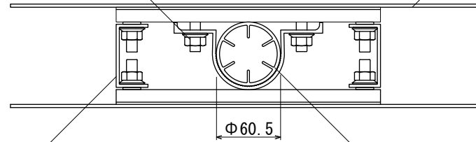
【平面図 S=1:5】
