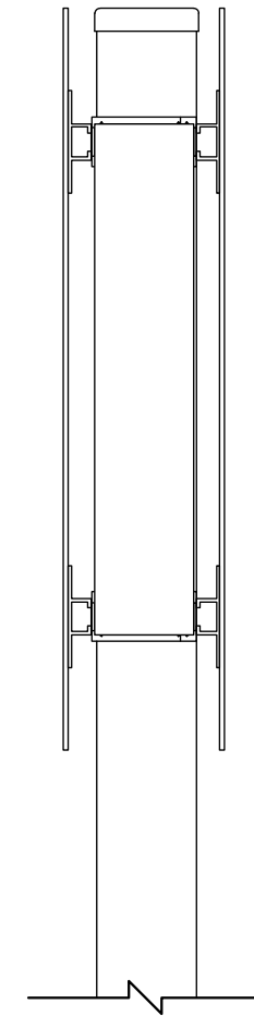
【側面図 S=1:5】
