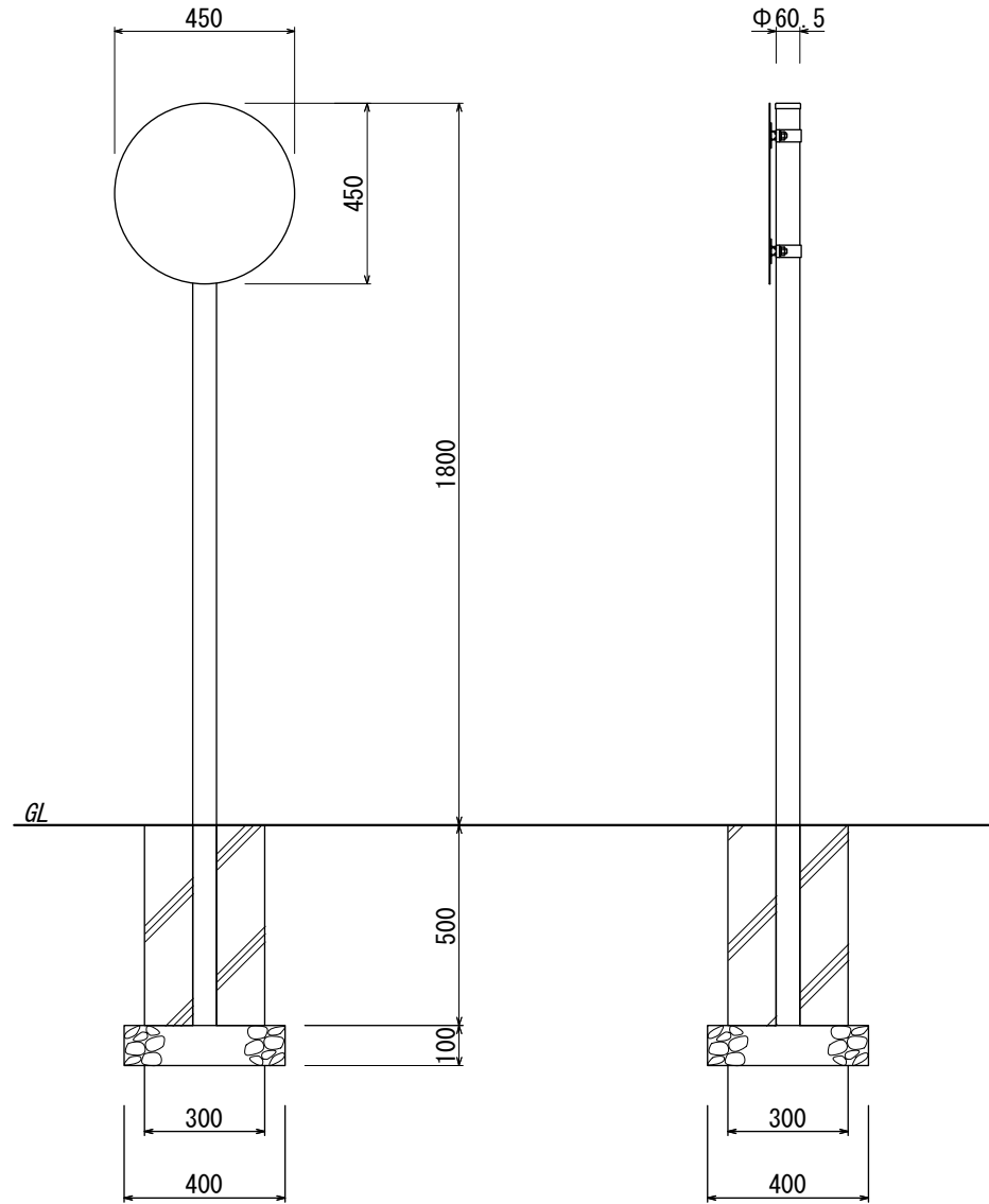
【正面図 S=1:20】
