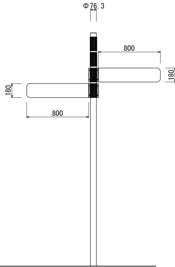
【側面図 S=1:30】
