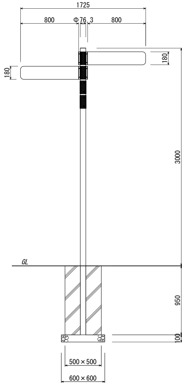
【正面図 S=1:30】
