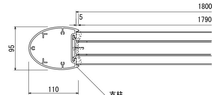
【平面図 S=1:5】
