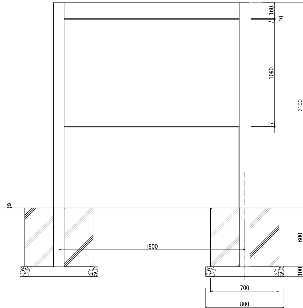
【正面図 S=1:20】
