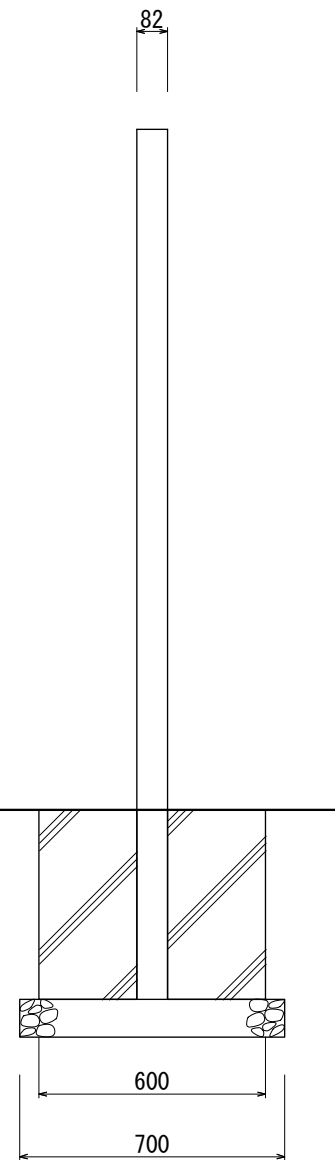
【側面図 S=1:20】
