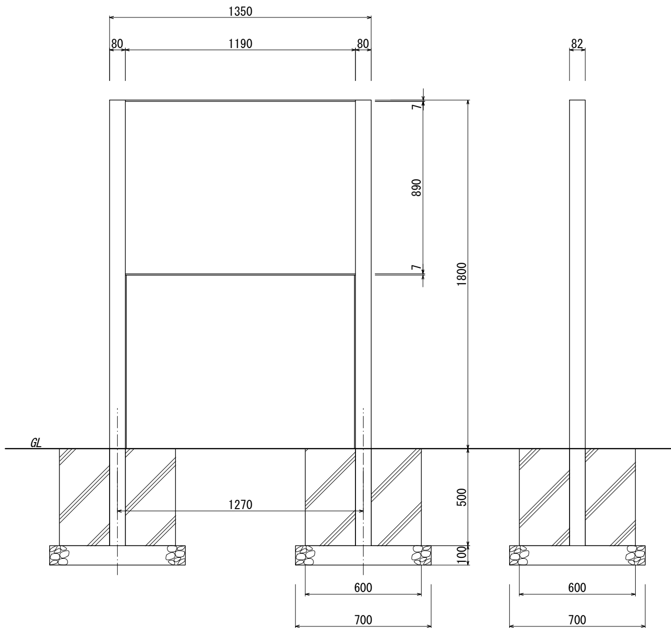
【正面図 S=1:20】
