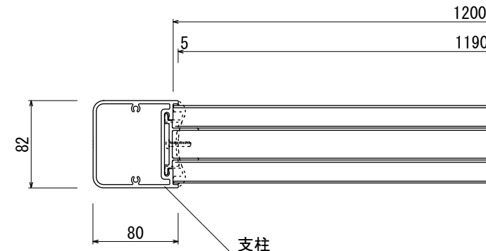
【平面図 S=1:5】
