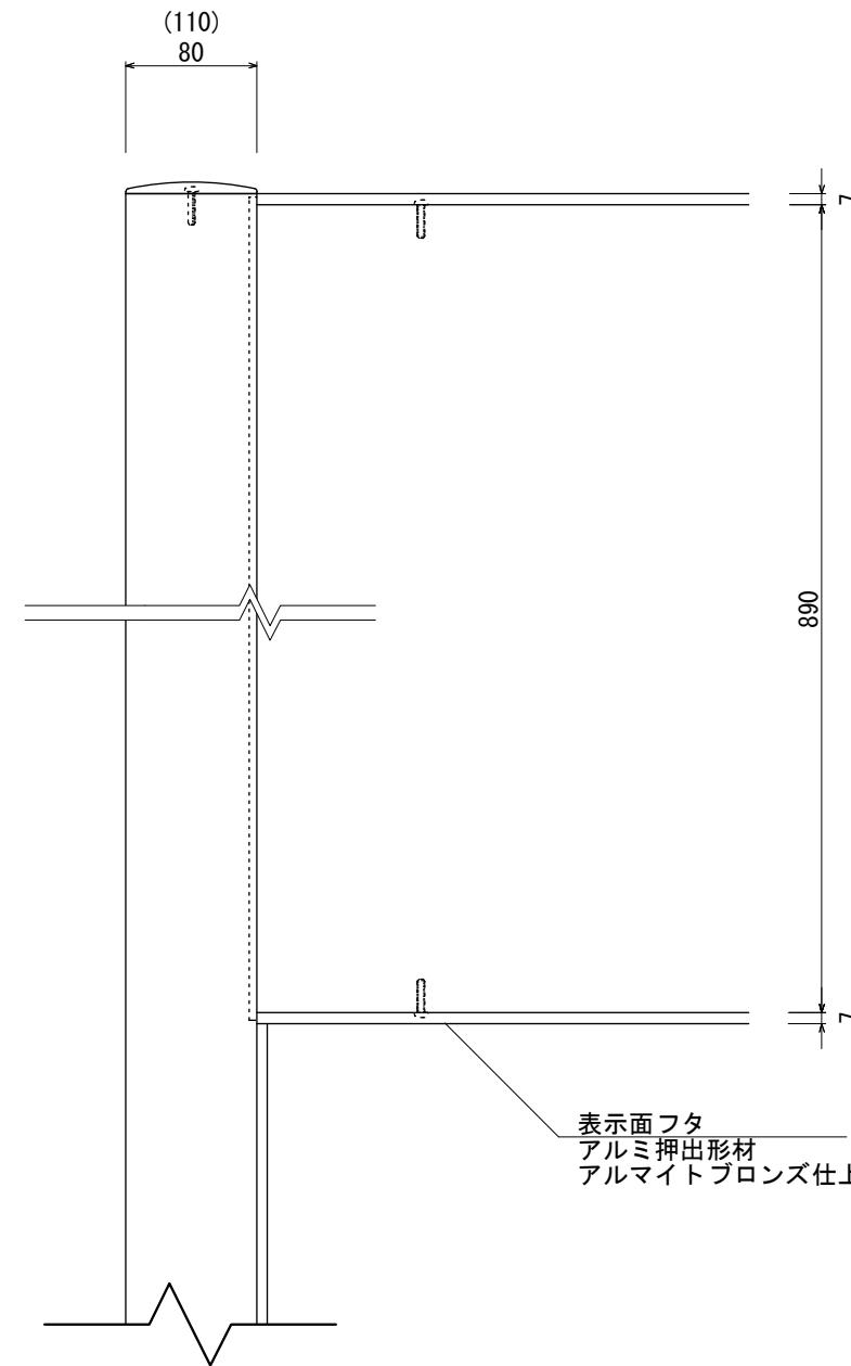
【正面図 S=1:5】
