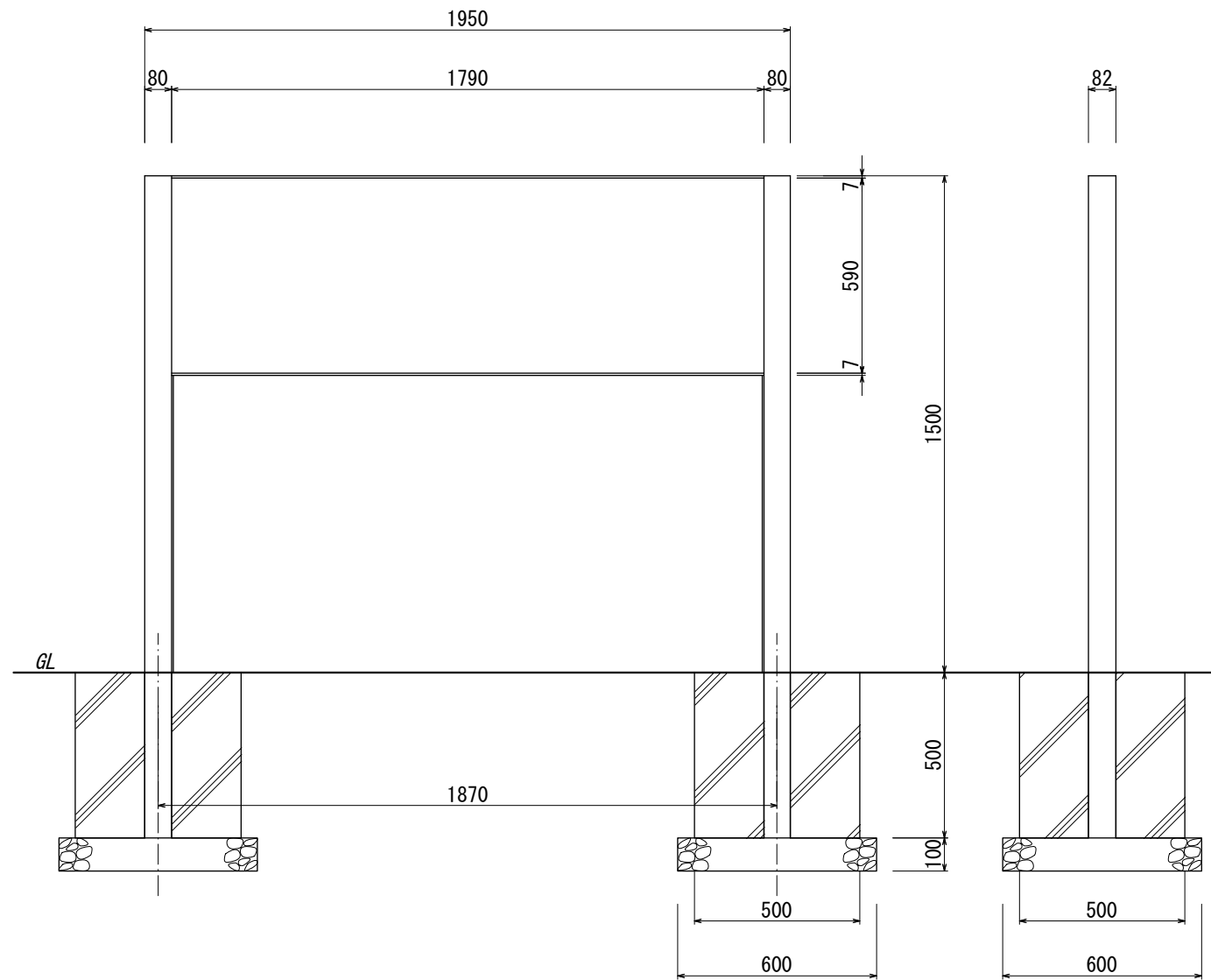
【正面図 S=1:20】
