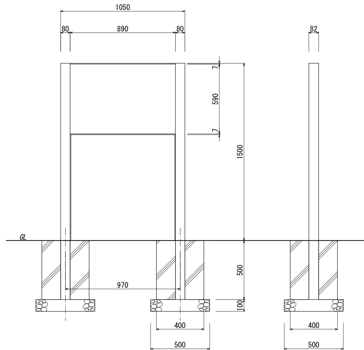
【正面図 S=1:20】
