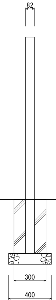
【側面図 S=1:20】
