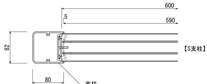
【平面図 S=1:5】
