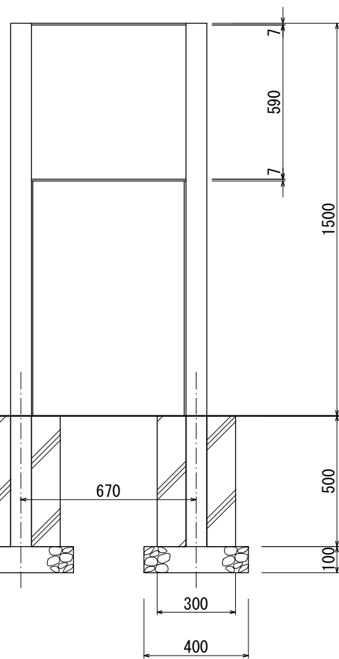
【正面図 S=1:20】
