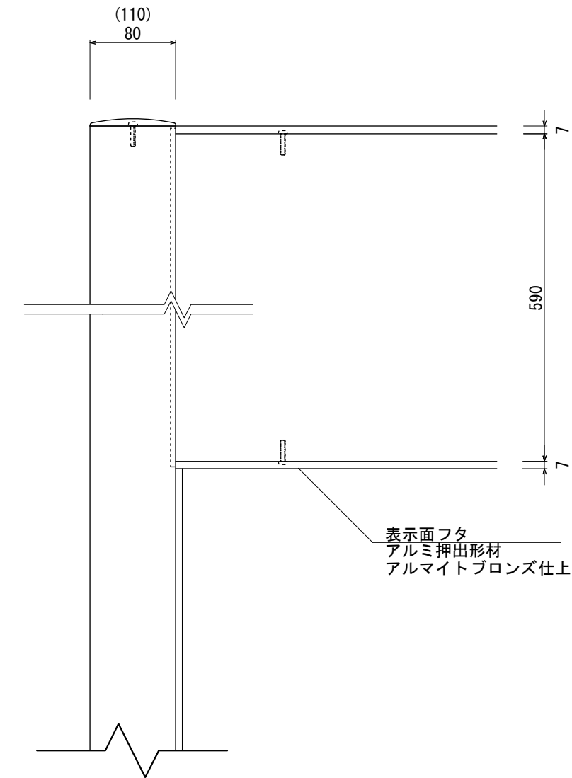
【正面図 S=1:5】
