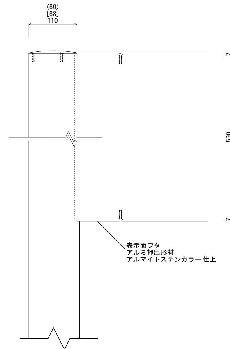
【正面図 S=1:5】
