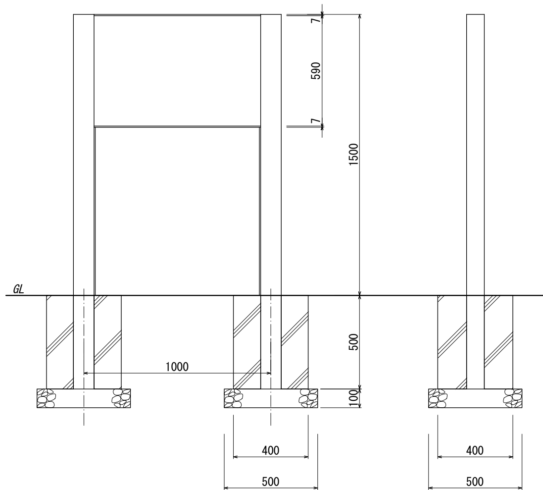
【正面図 S=1:20】
