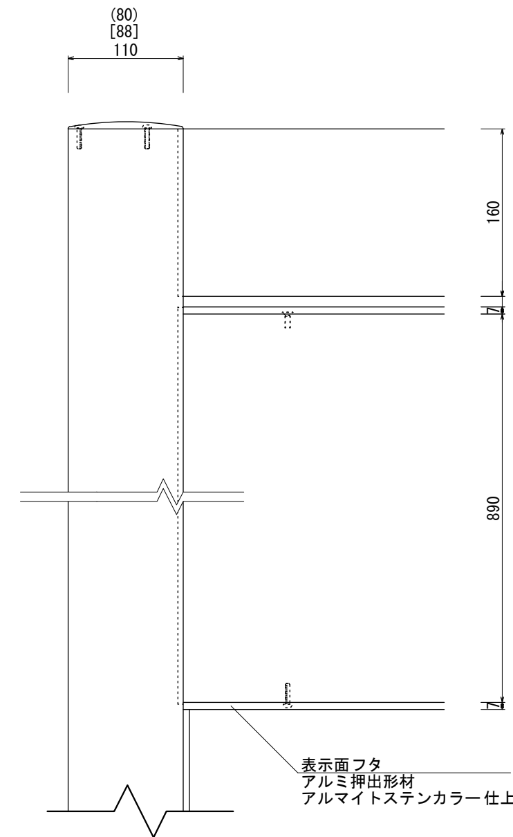
【正面図 S=1:5】
