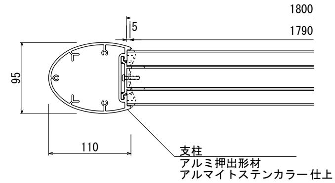
【平面図 S=1:5】
