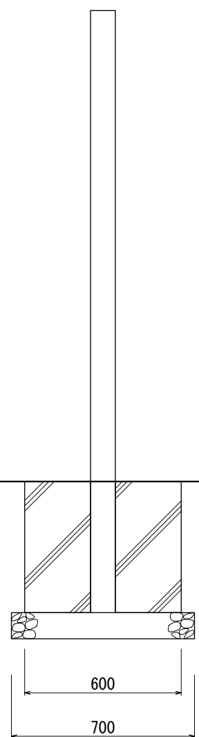
【側面図 S=1:20】
