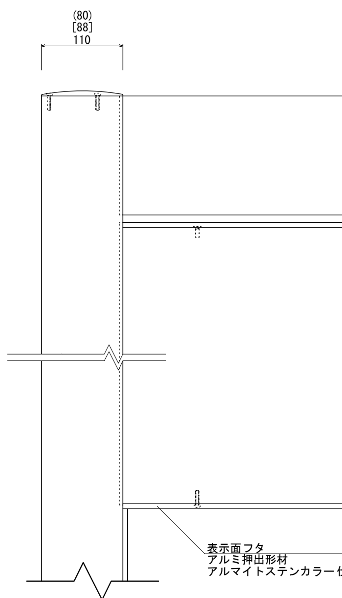
【正面図 S=1:5】
