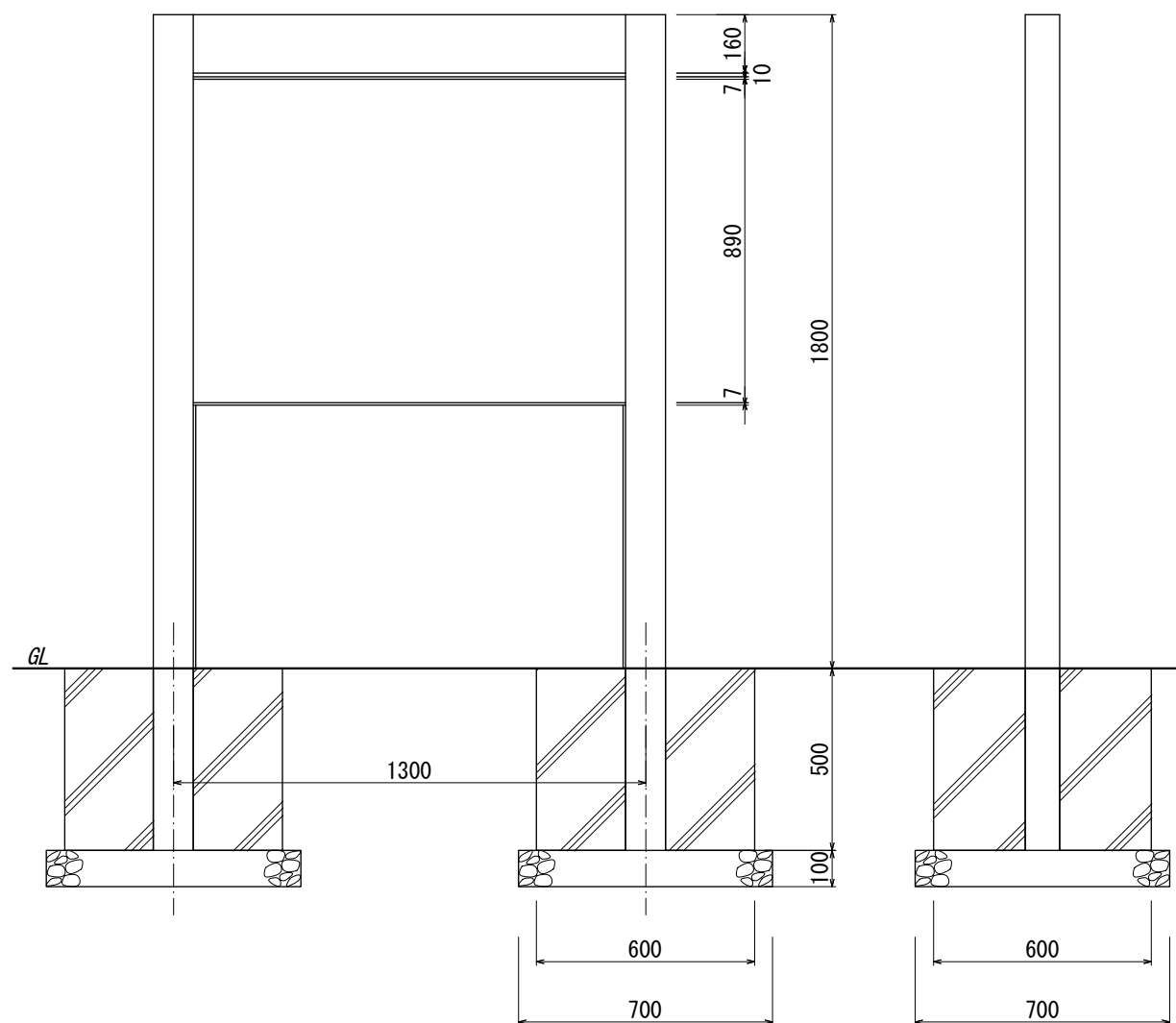
【正面図 S=1:20】
