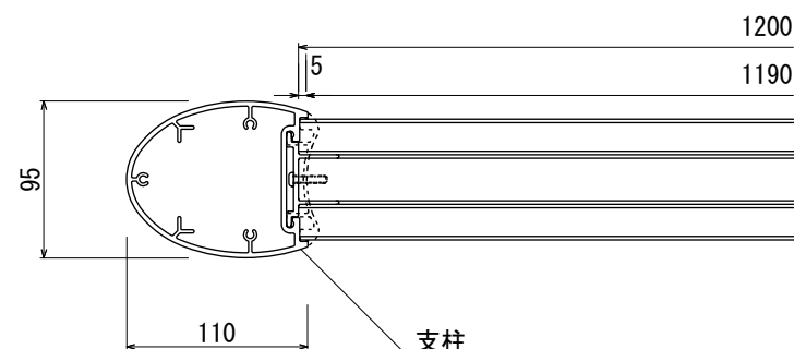
【平面図 S=1:5】
