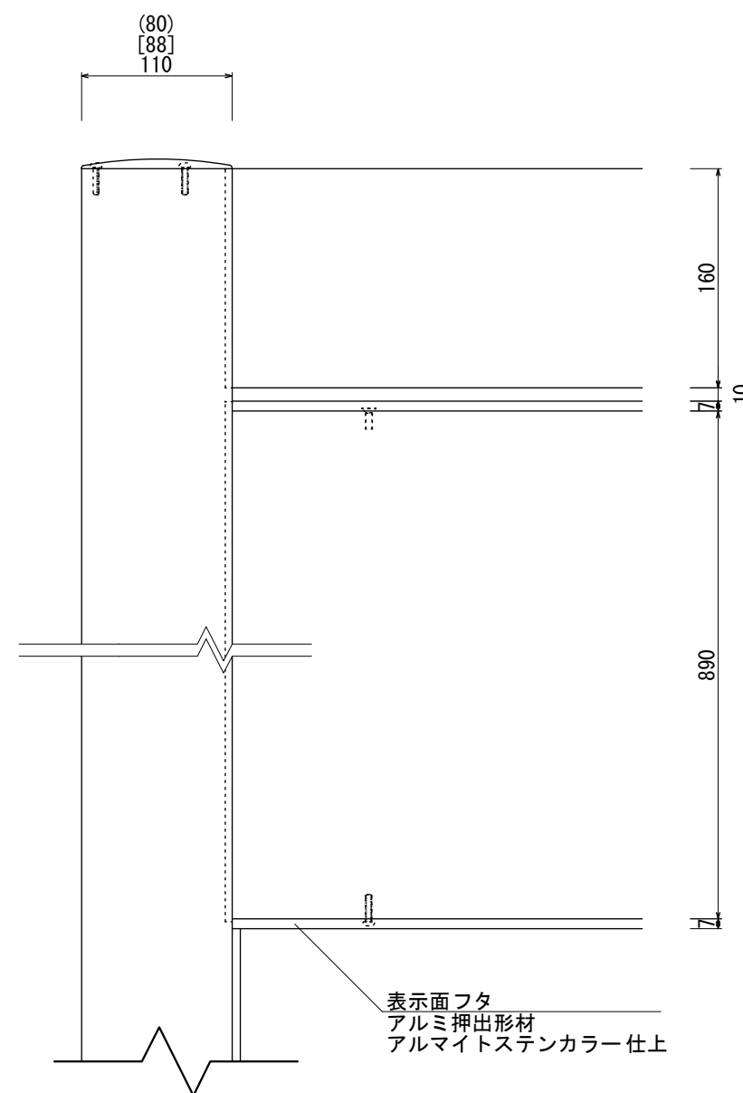
【正面図 S=1:5】
