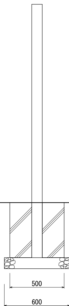
【側面図 S=1:20】
