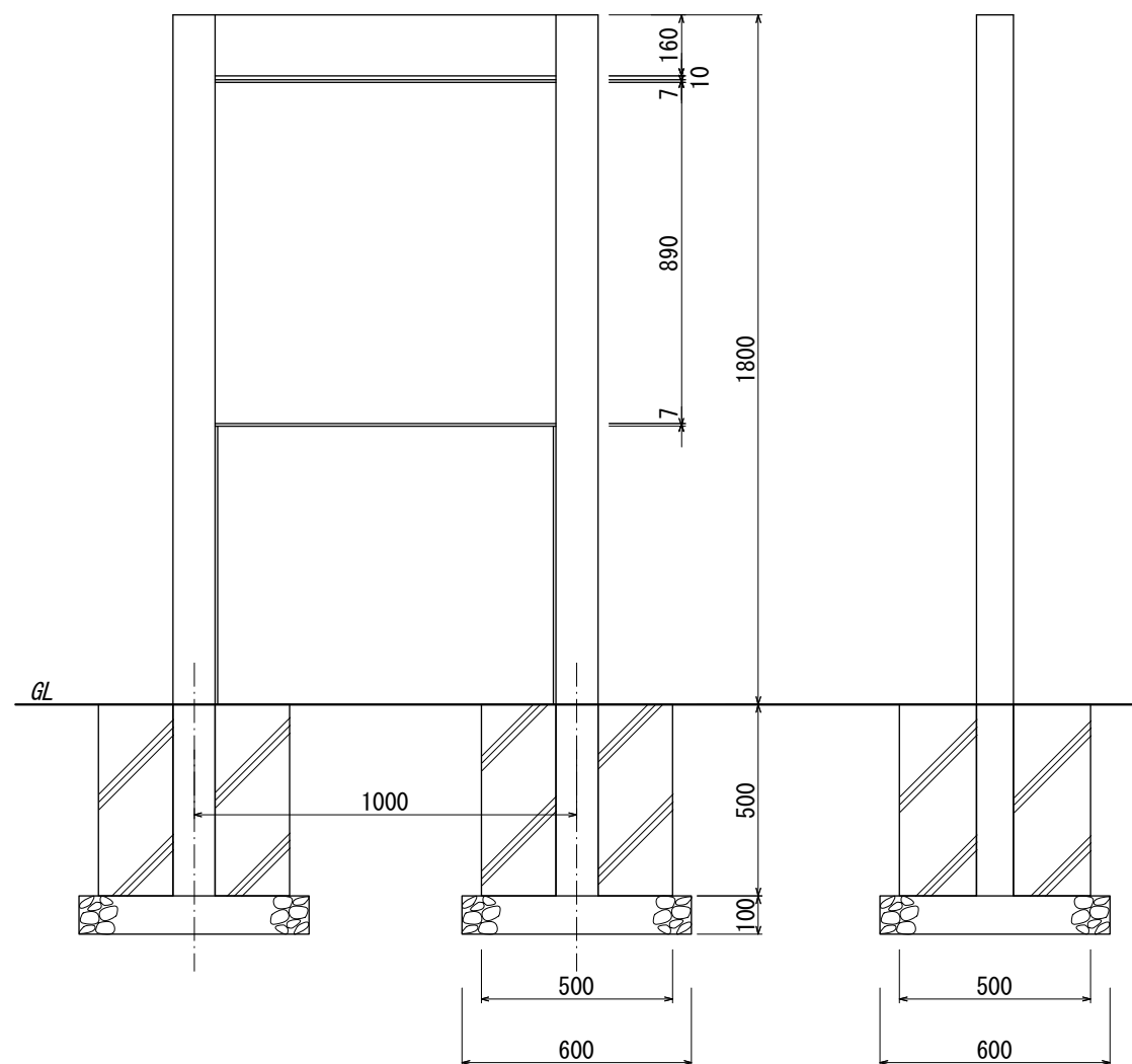
【正面図 S=1:20】
