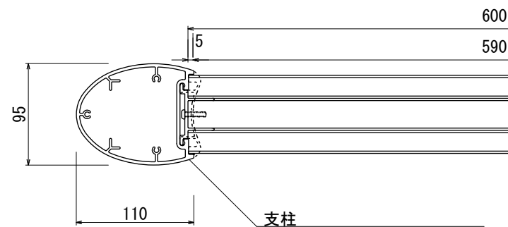
【平面図 S=1:5】
