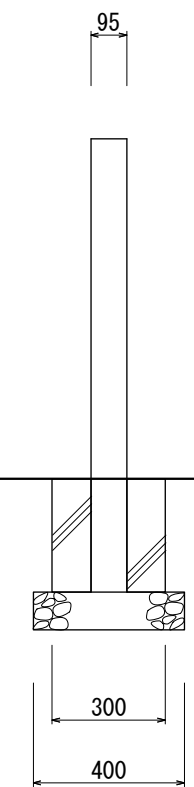
【側面図 S=1:20】
