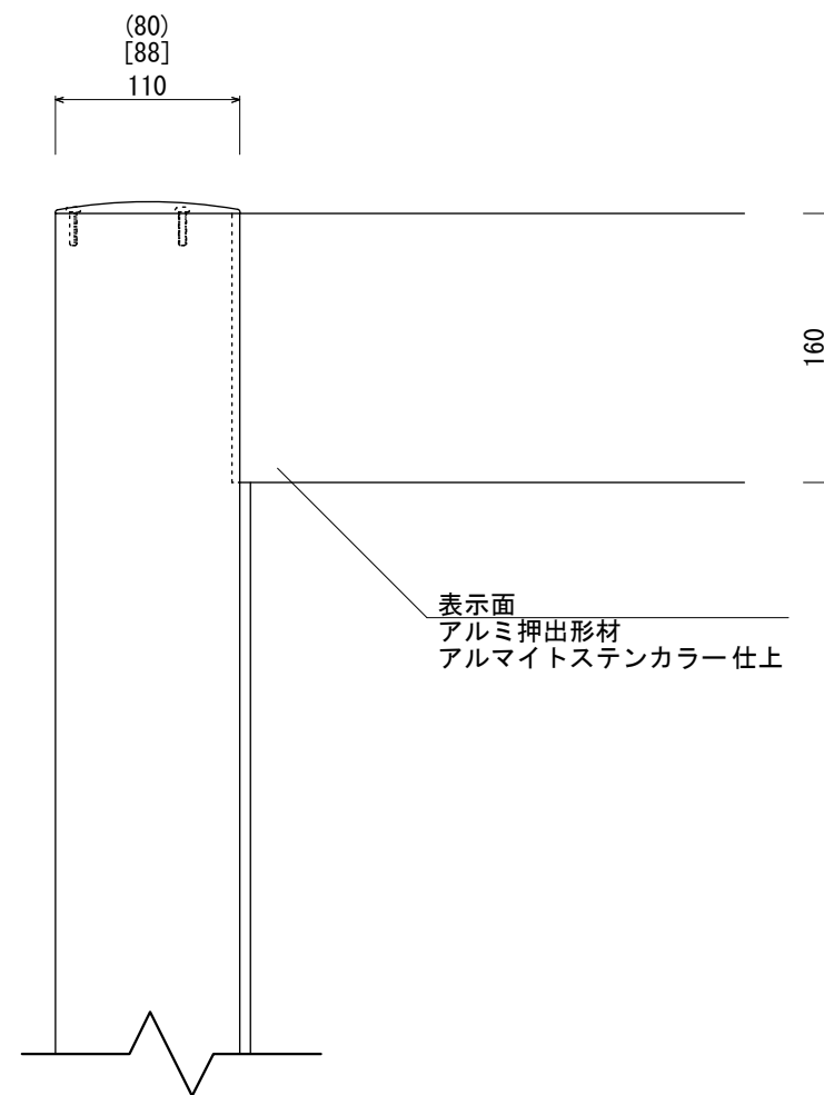
【正面図 S=1:5】
