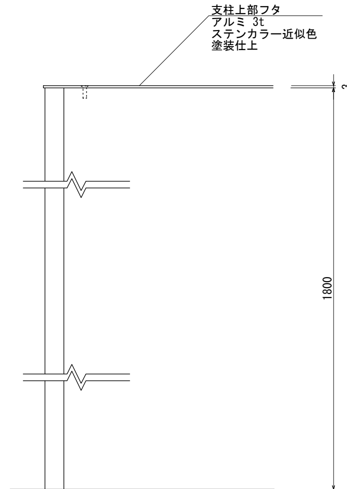
【正面図 S=1:5】
