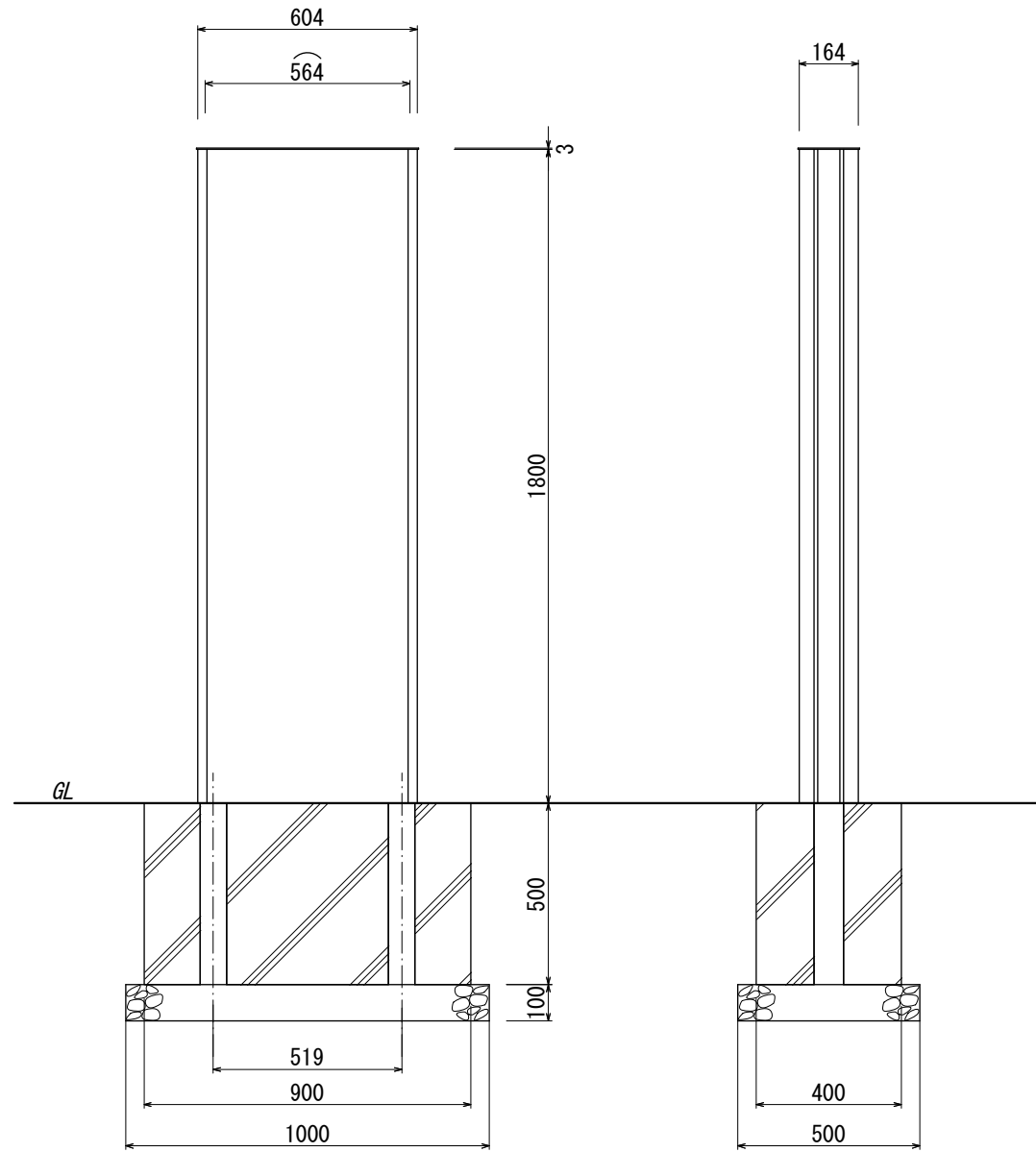
【正面図 S=1:20】
