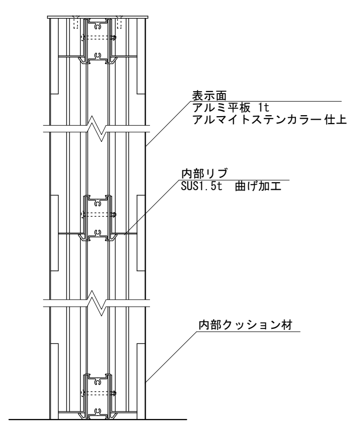
【側断面図 S=1:5】
