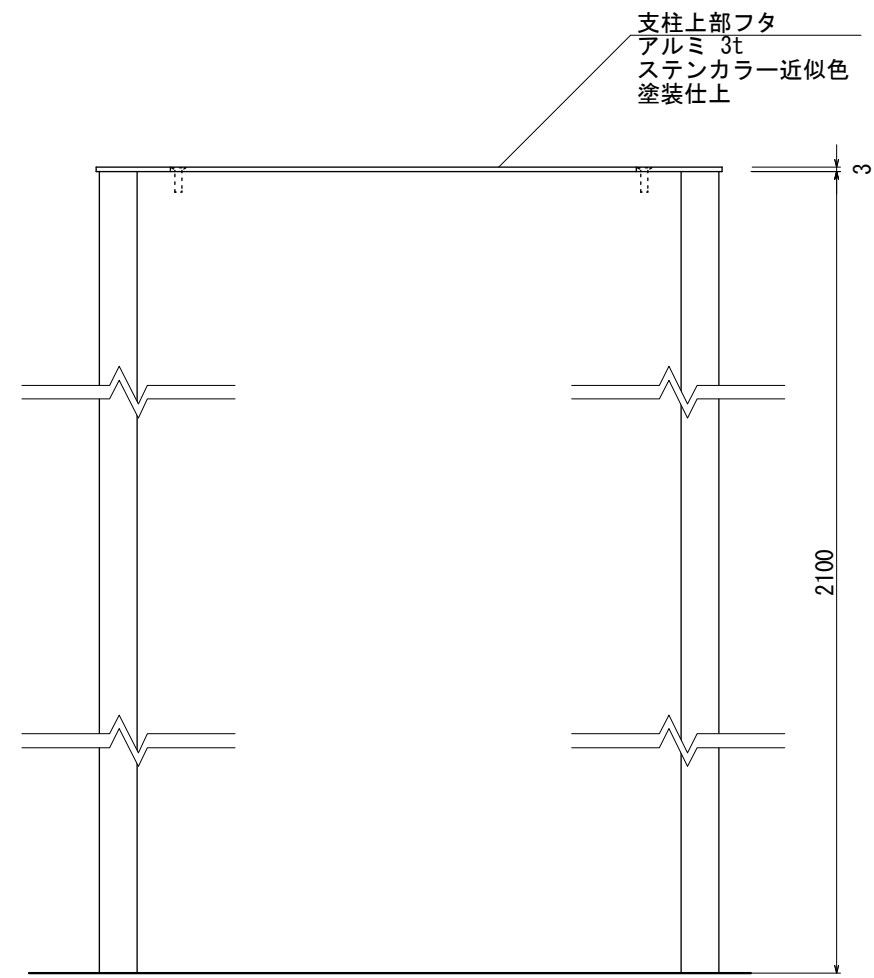
【正面図 S=1:5】
