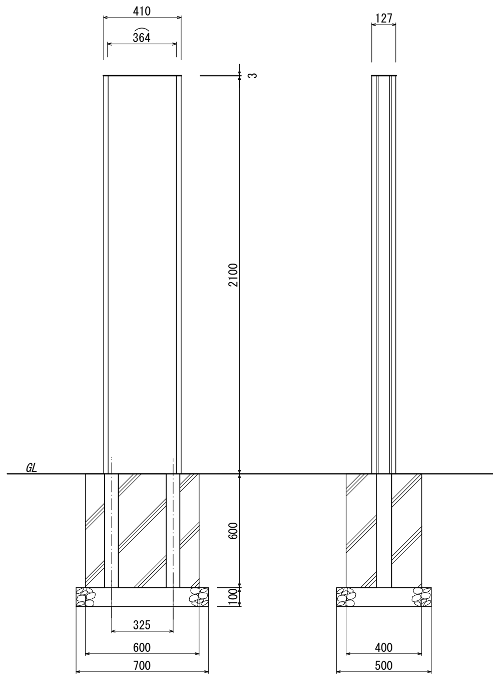
【正面図 S=1:20】
