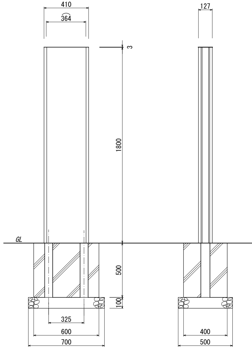
【正面図 S=1:20】
