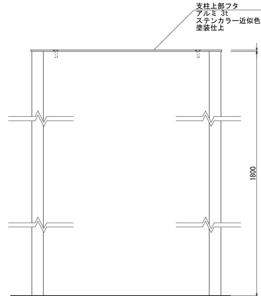
【正面図 S=1:5】
