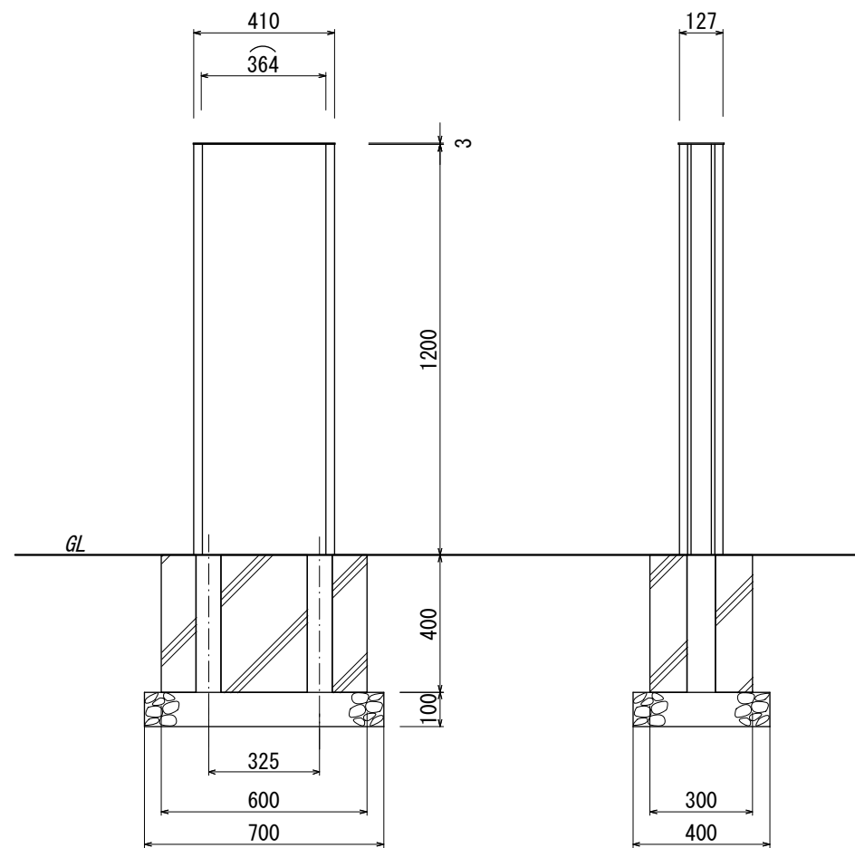
【正面図 S=1:20】
