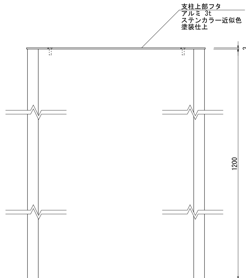
【正面図 S=1:5】
