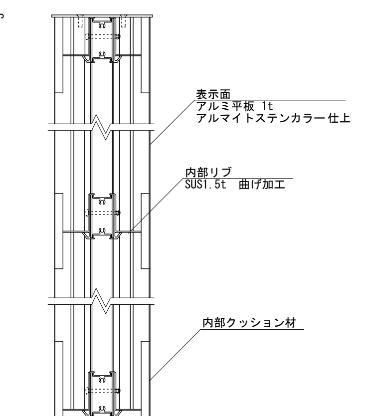
【側断面図 S=1:5】
