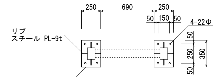
【ベース詳細図 S=1:30】
