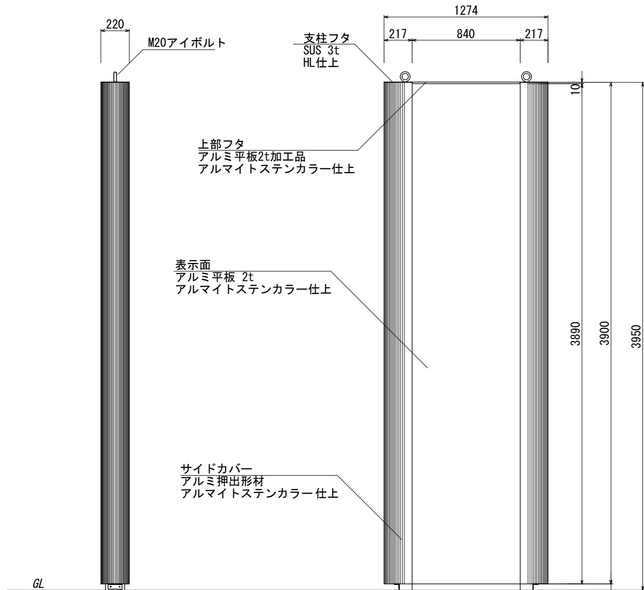
【側面図 S=1:30】
