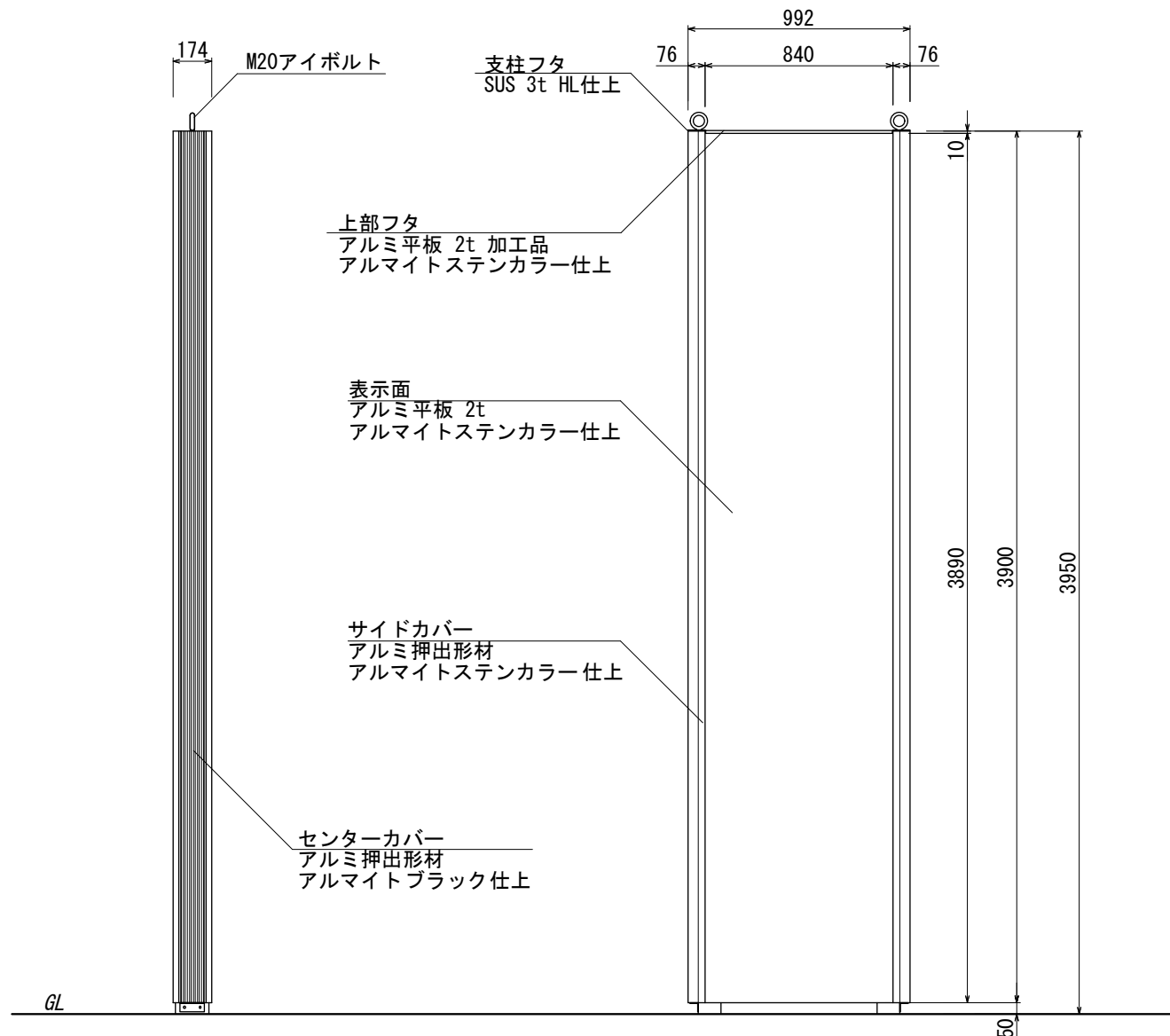
【側面図 S=1:30】
