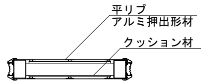
【断面図 S=1:30】
