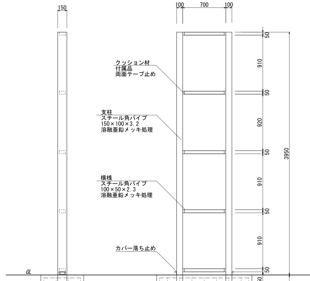
【鉄骨断面図 S=1:30】
