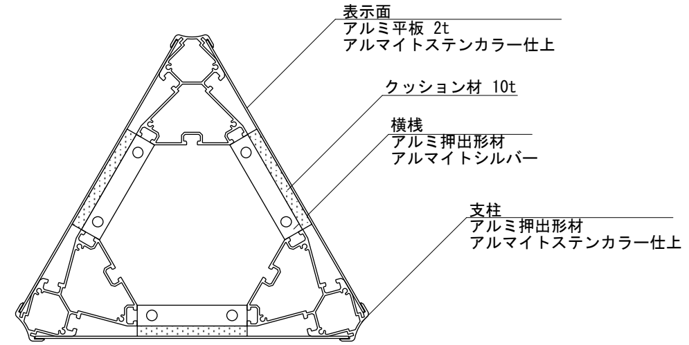
【断面図 S=1:5】
