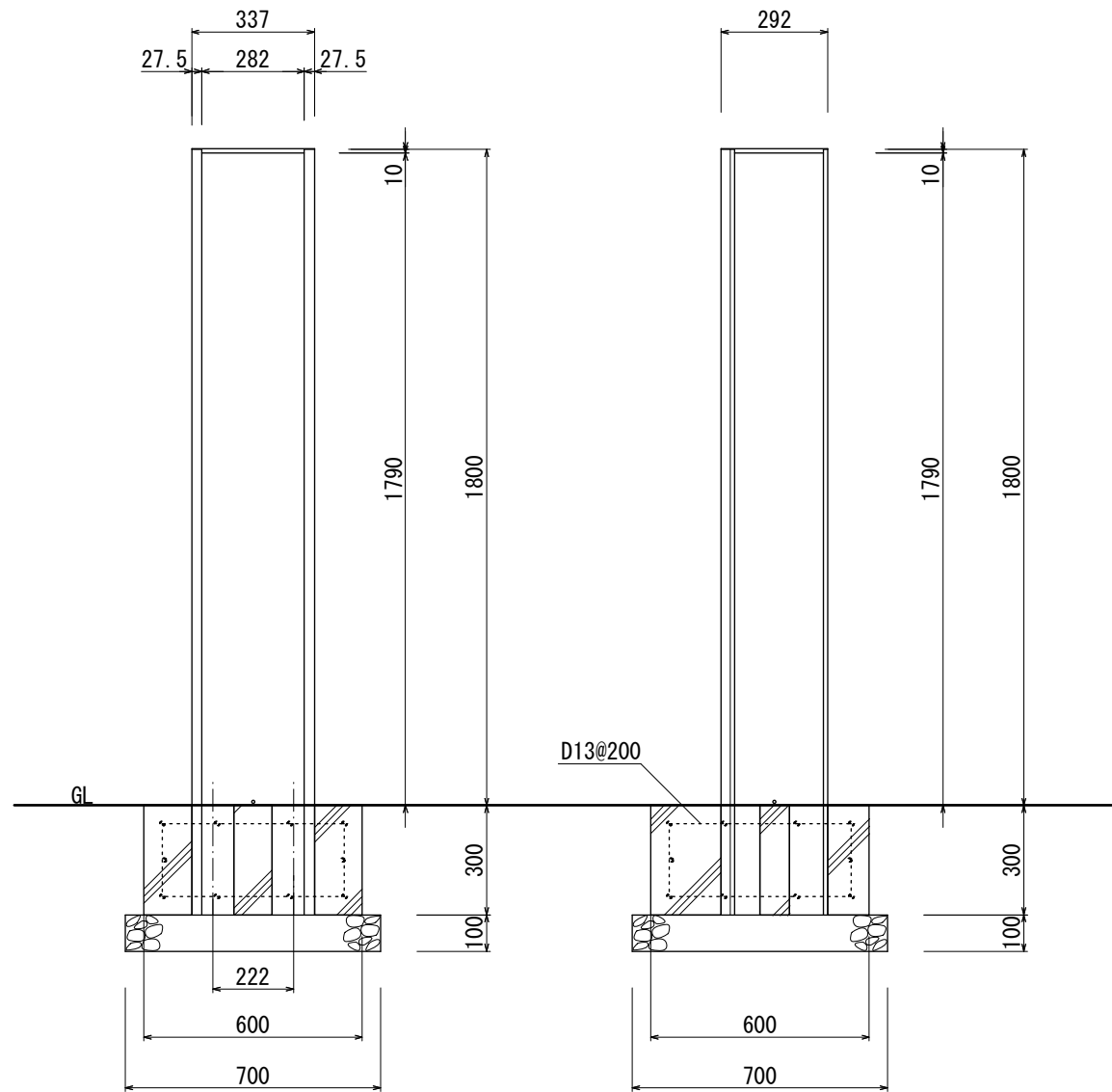
【正面図 S=1:20】
