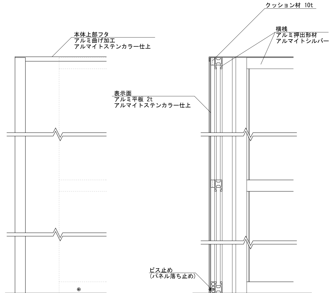
【断面図 S=1:5】
