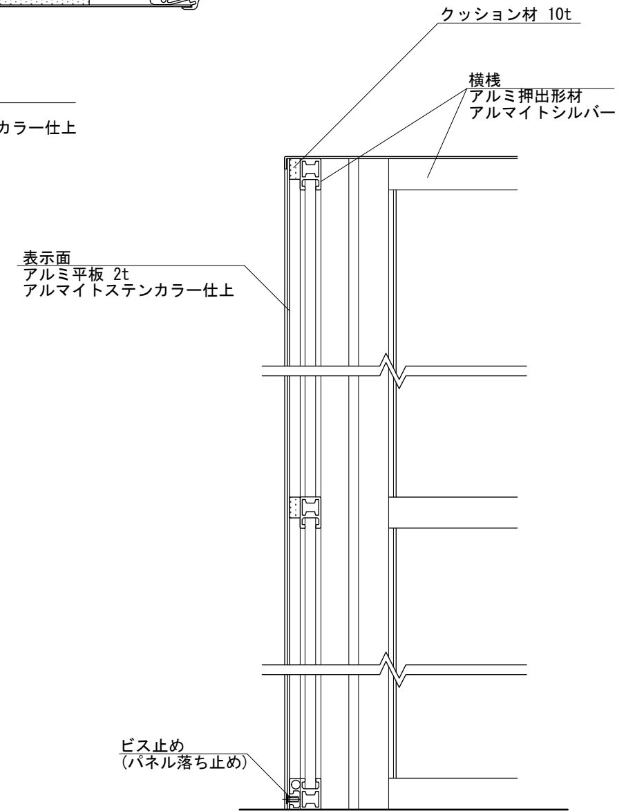
【断面図 S=1:5】
