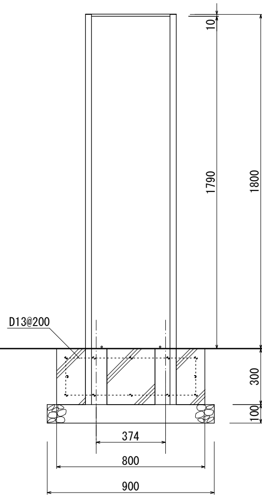
【側面図 S=1:20】
