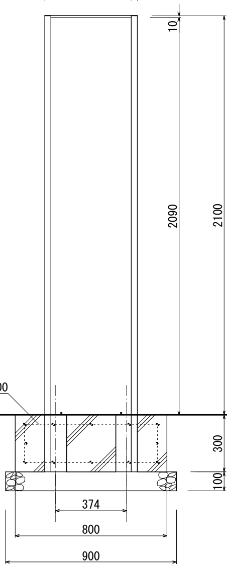
【側面図 S=1:20】
