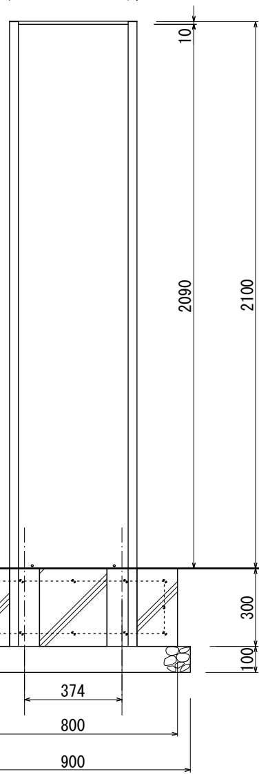
【正面図 S=1:20】
