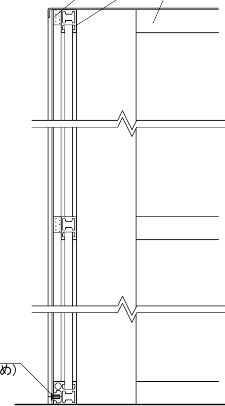
【断面図 S=1:5】
