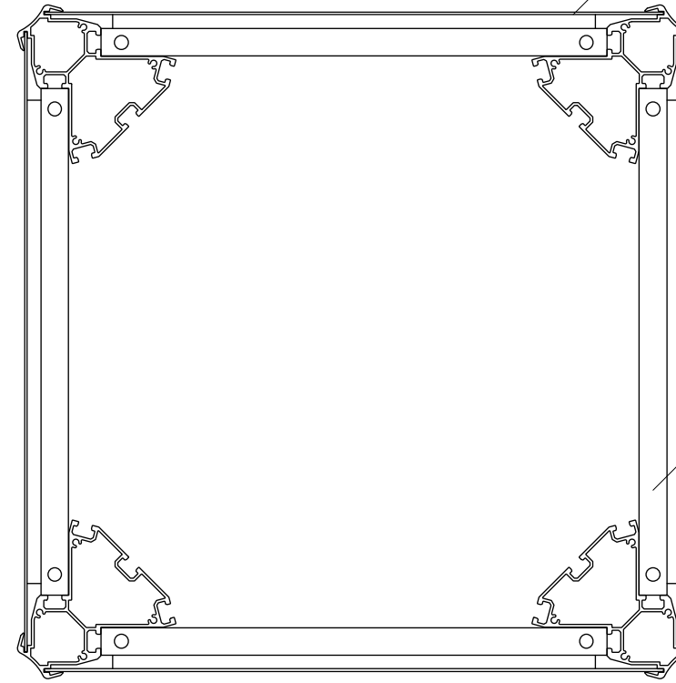
【断面図 S=1:5】
