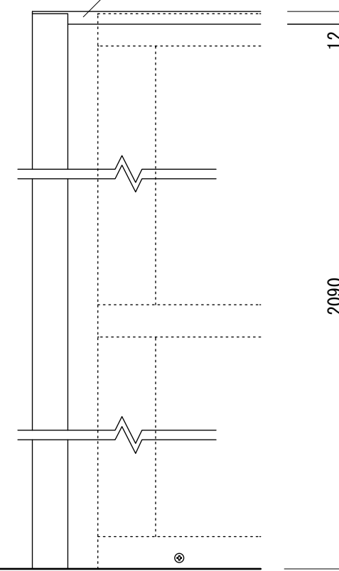
【正面図 S=1:5】
