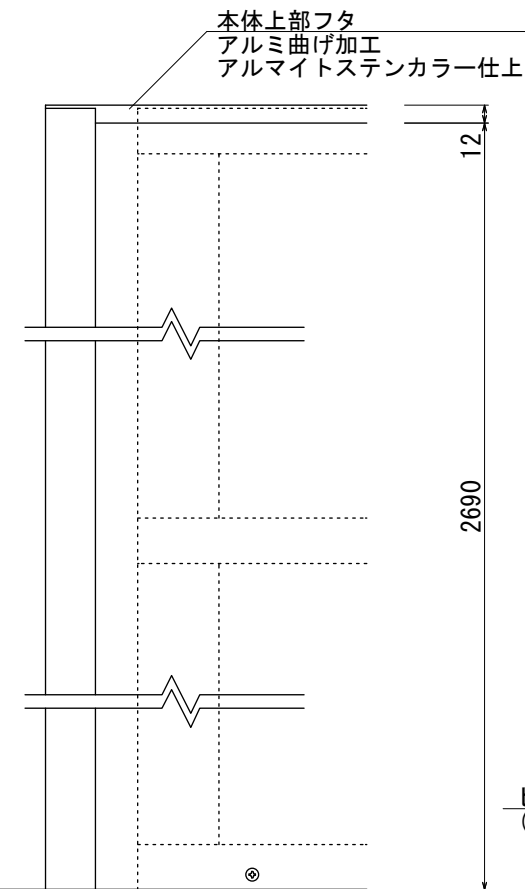
【正面図 S=1:5】
