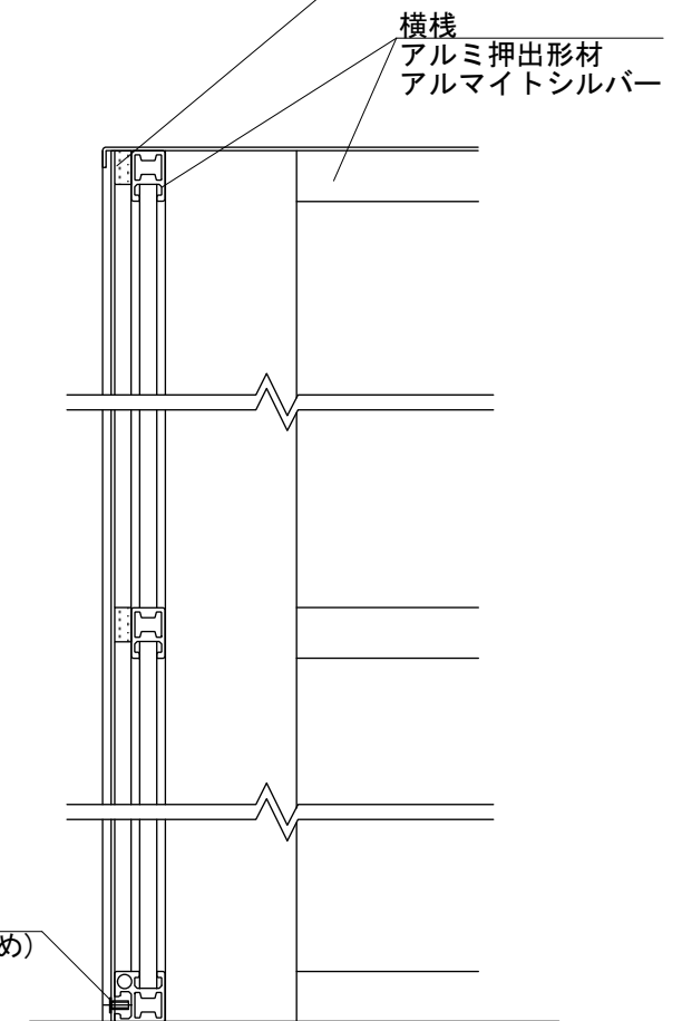
【断面図 S=1:5】
