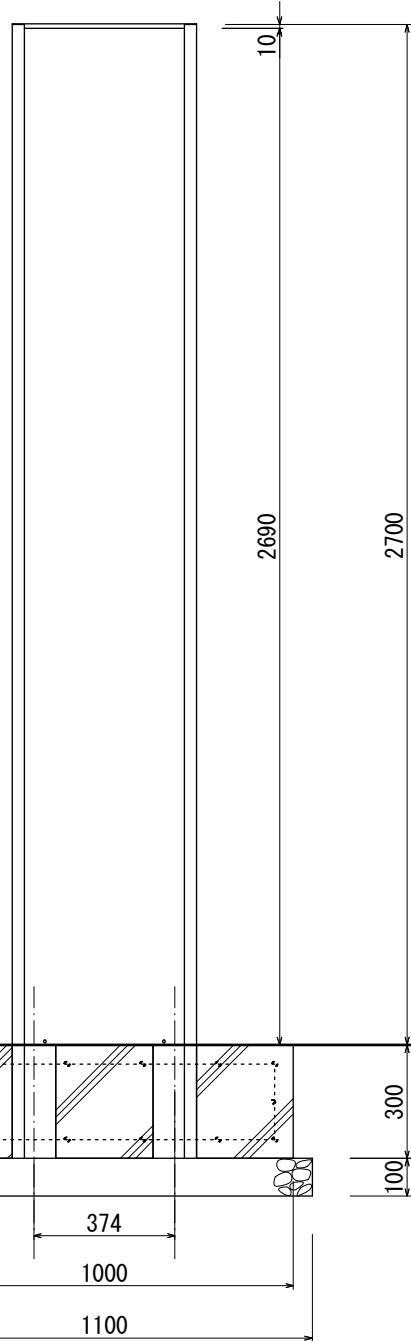
【正面図 S=1:20】
