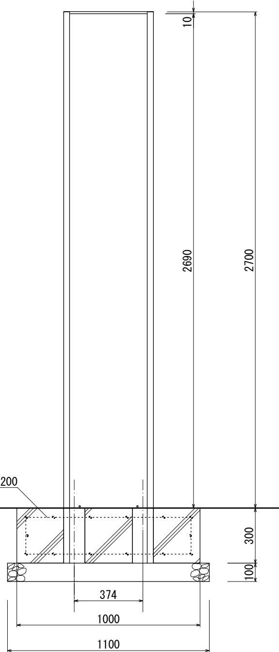
【側面図 S=1:20】
