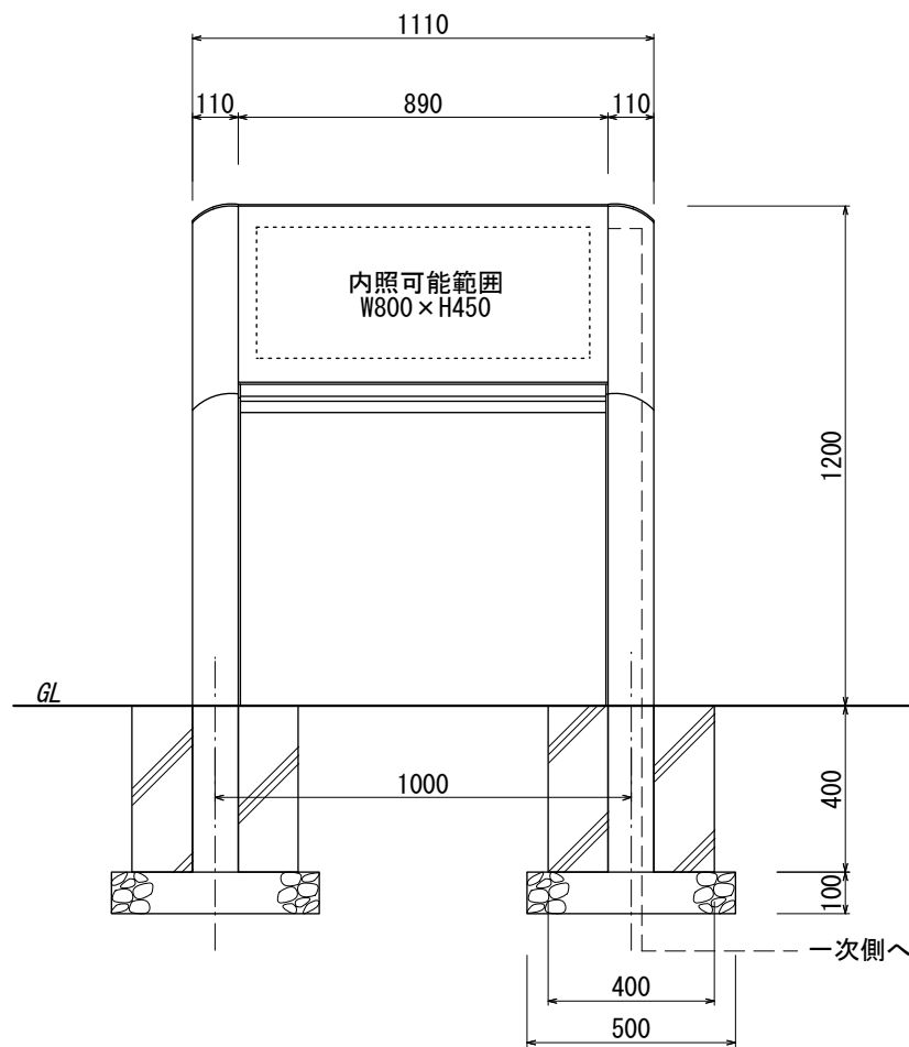
【正面図 S=1:20】
