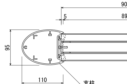
【平面図 S=1:5】
