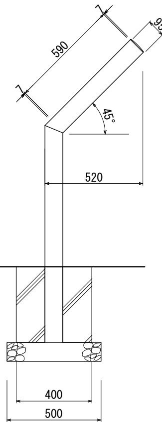
【側面図 S=1:20】
