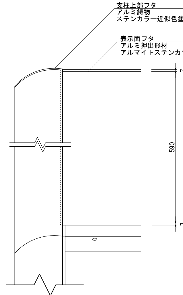
【正面図 S=1:5】
