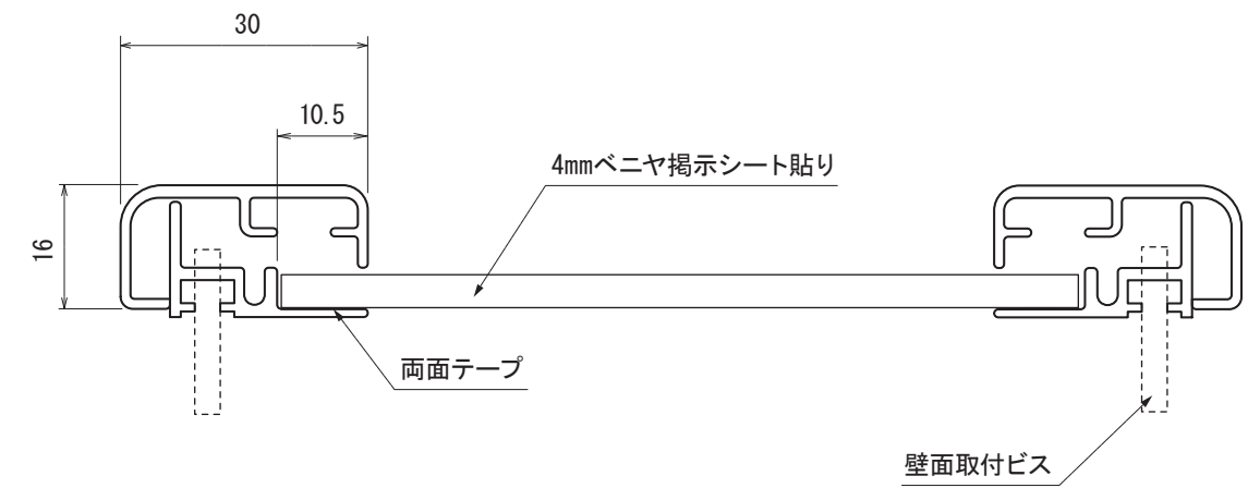
断面A-A'
