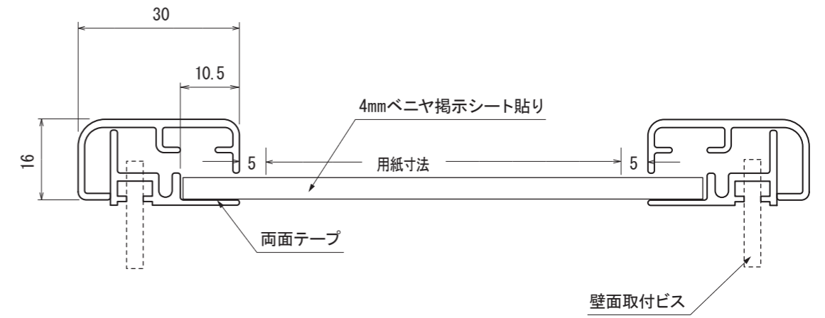
断面A-A'
