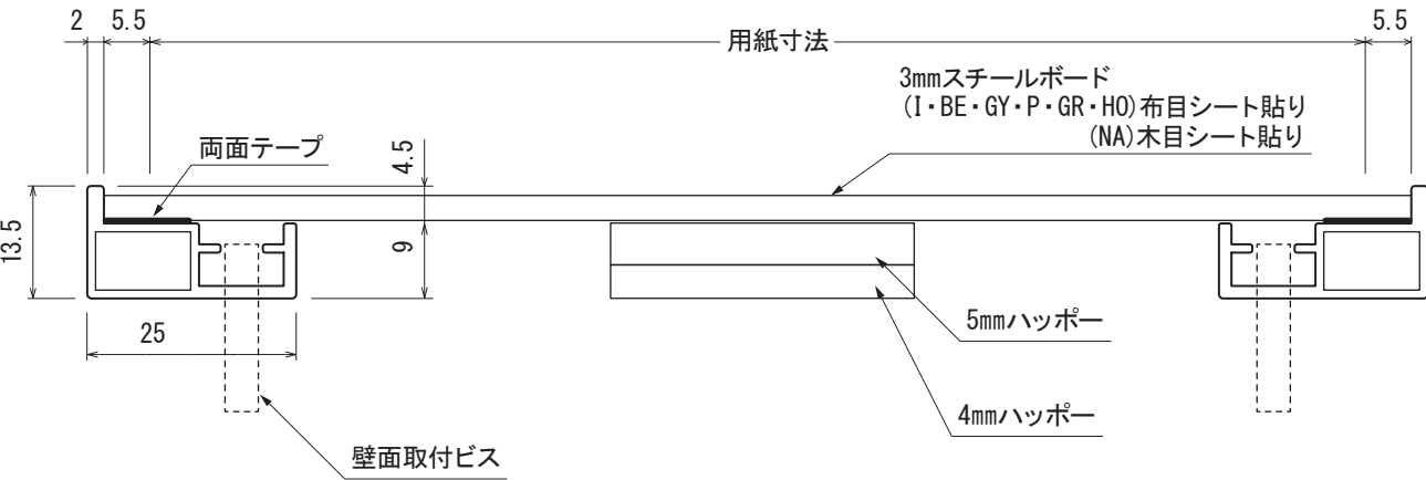
断面A-A'
