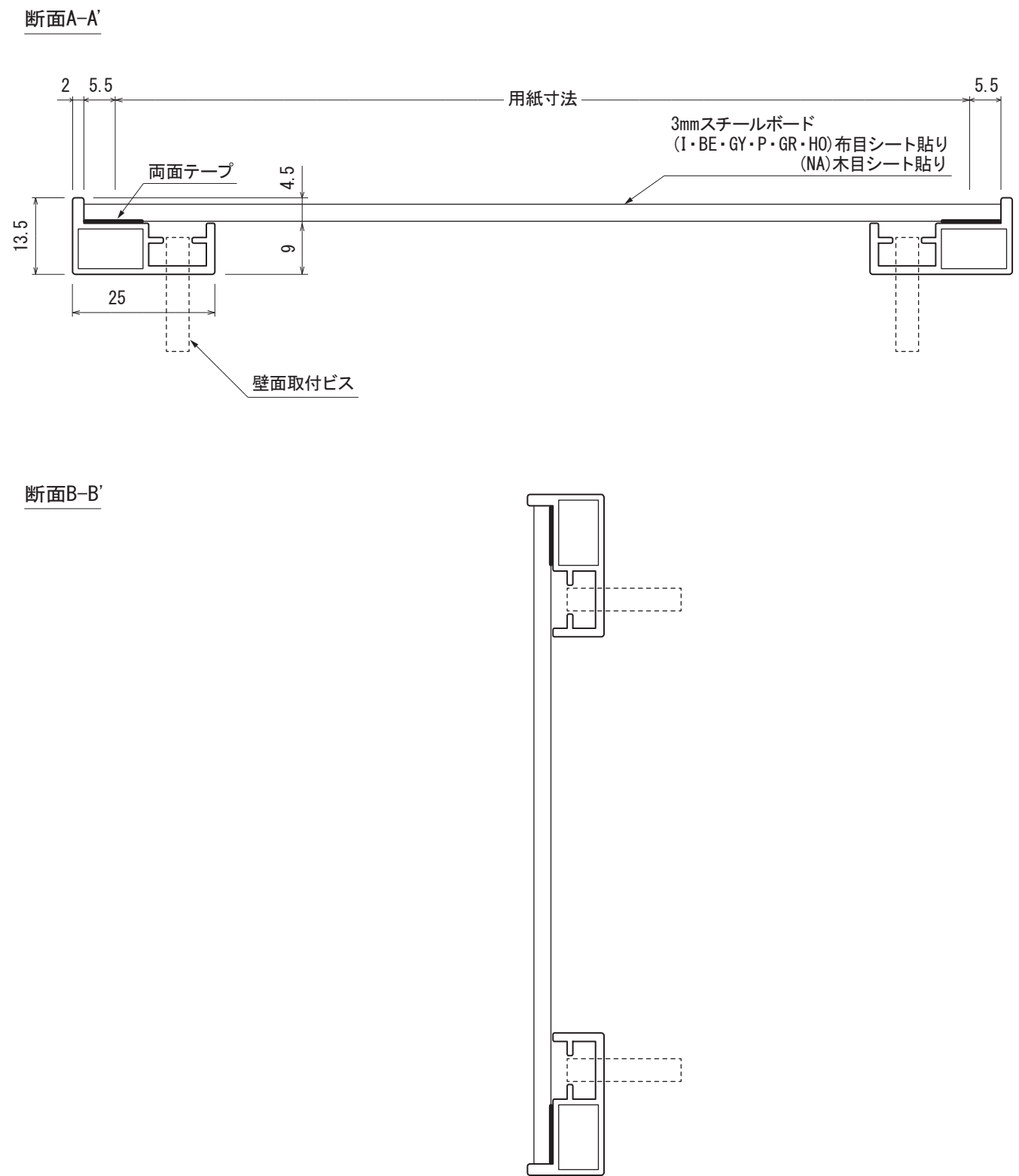
断面詳細図 (S=1/1)
