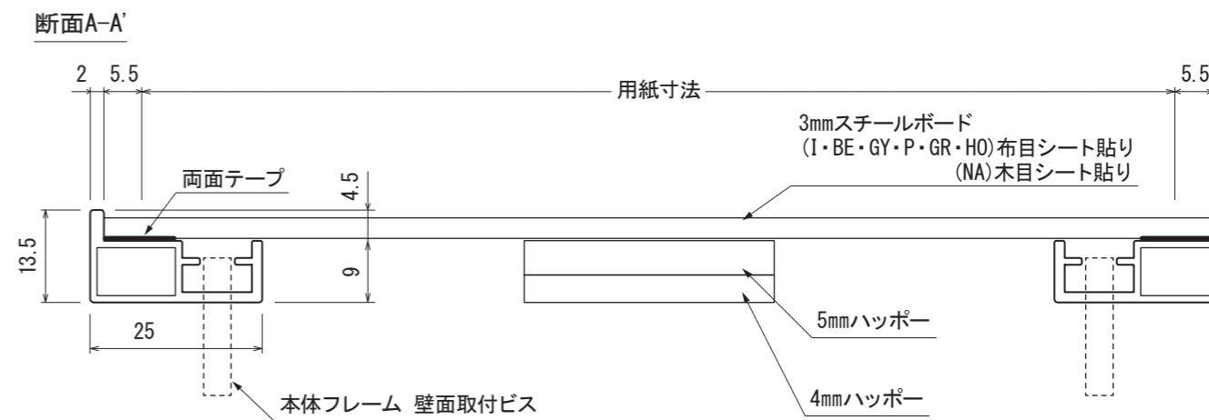
断面詳細図 (S=1/1)
