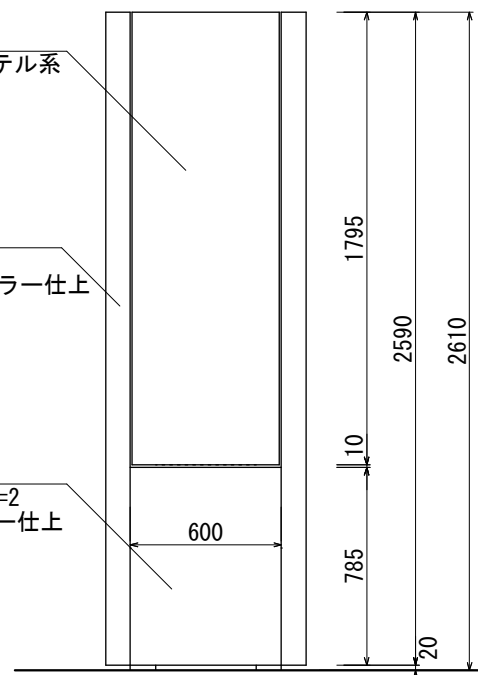
【正面図 S=1:30】
