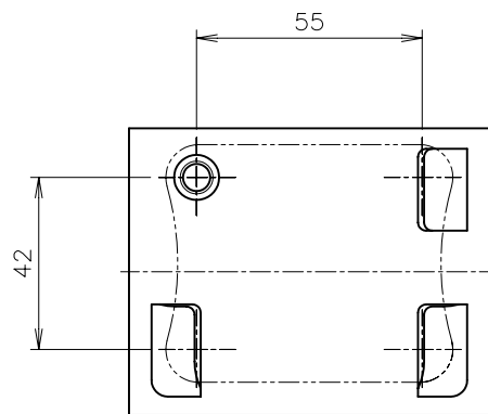
取付部詳細図 (S=1:2)
